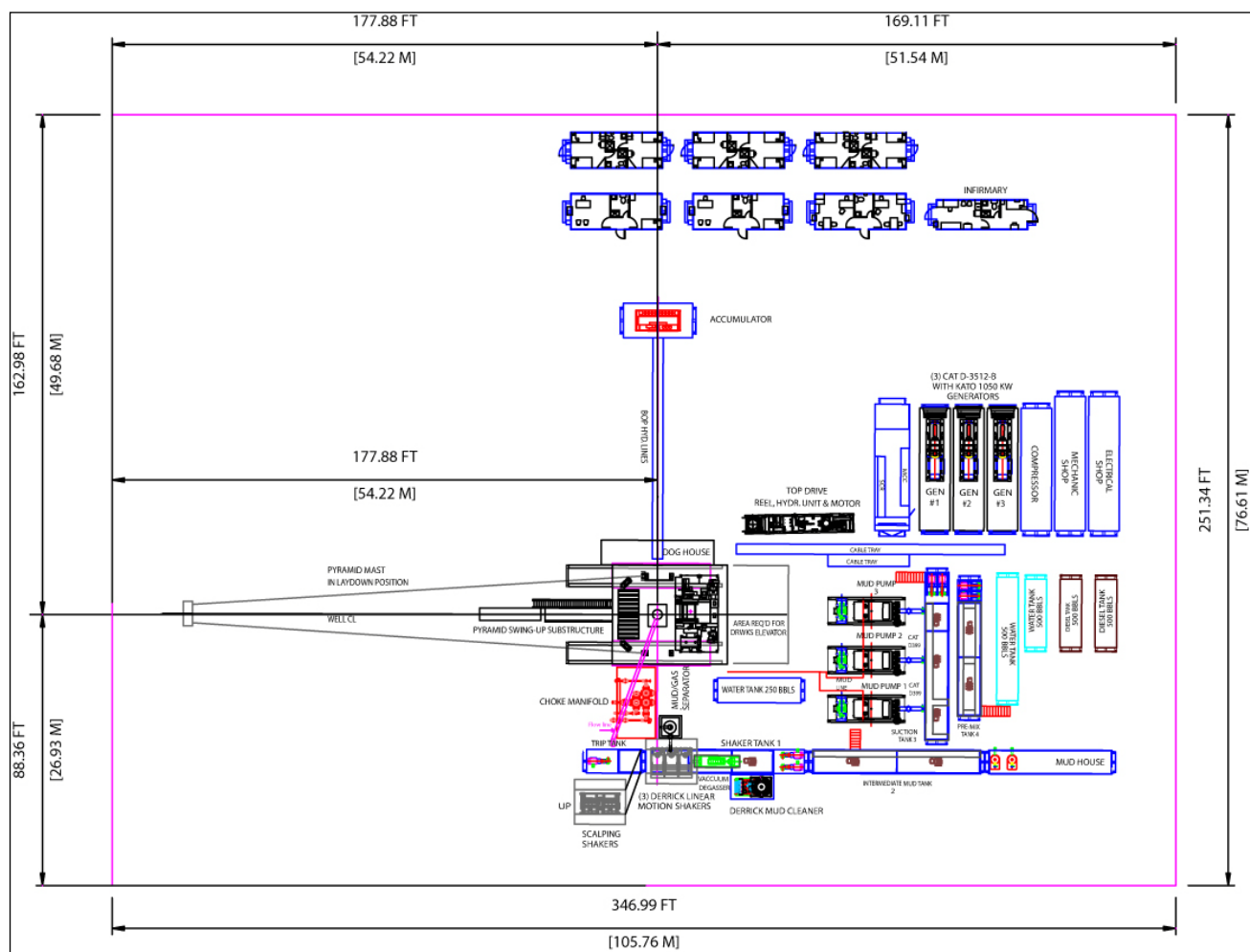
Figura 24. Diseño del arreglo de un equipo de perforación de 2.000 HP
