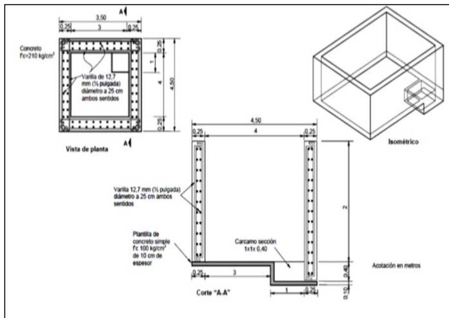
Figura 23. Diseño del contra pozo.
