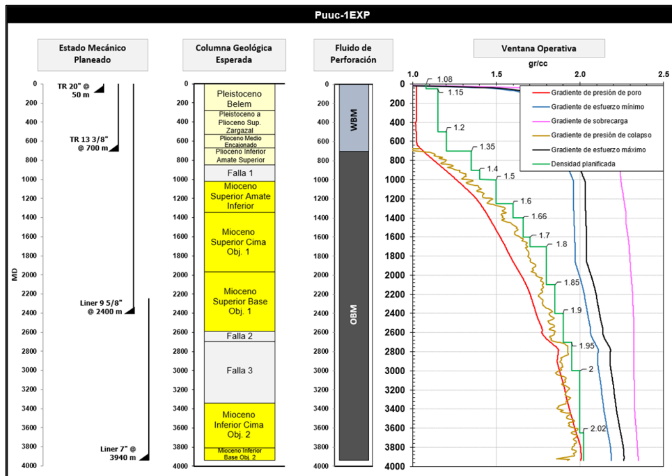
Figura 2. Estado mecánico del pozo
