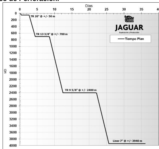
Gráfica de tiempo Vs. Profundidad
