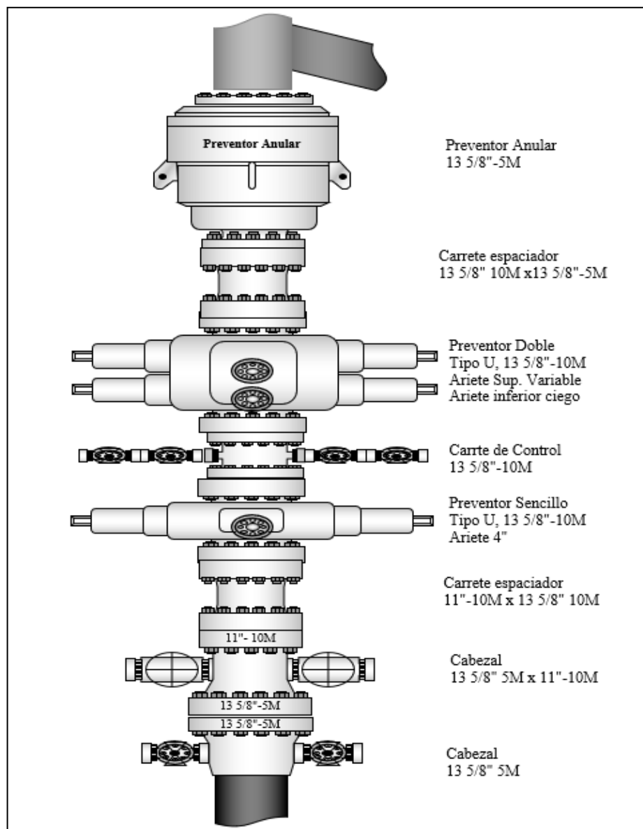
Figura 27. Arreglo de Preventor Esférico de 13 5/8" 5M con Aríete Superior Variable y Aríete Inferior Ciego, Carrete de Control de 13 5/8" 10M con Salidas Laterales de 3 1/16" 10M y Válvula Mecánica de 3 1/8", Brida de 3 1/16", Preventor Sencillo de 13 5/8" 10M y Cabezal 11" 10M para la Etapa 8 1/2"
