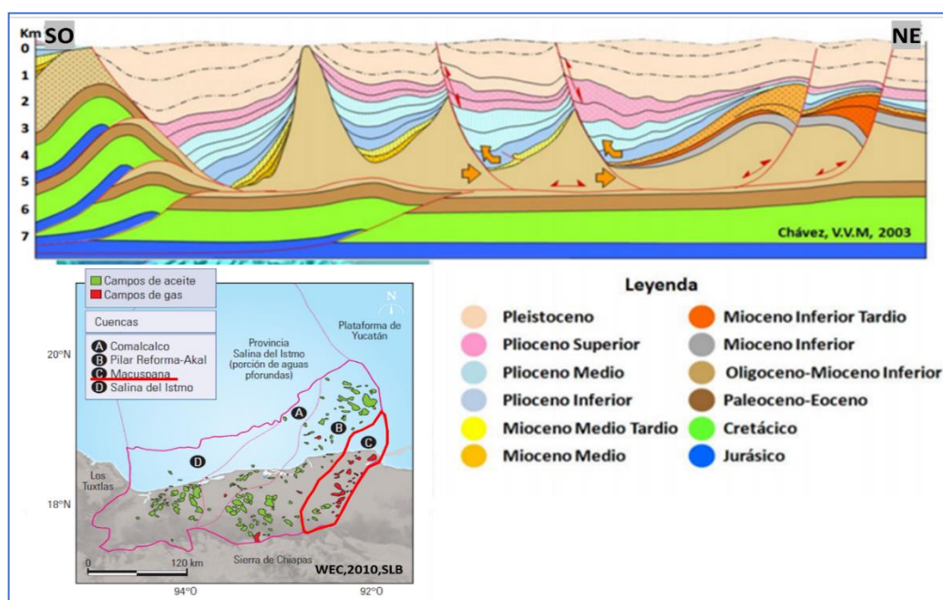
Figura 6. Sección estructural de la cuenca de Macuspana.
