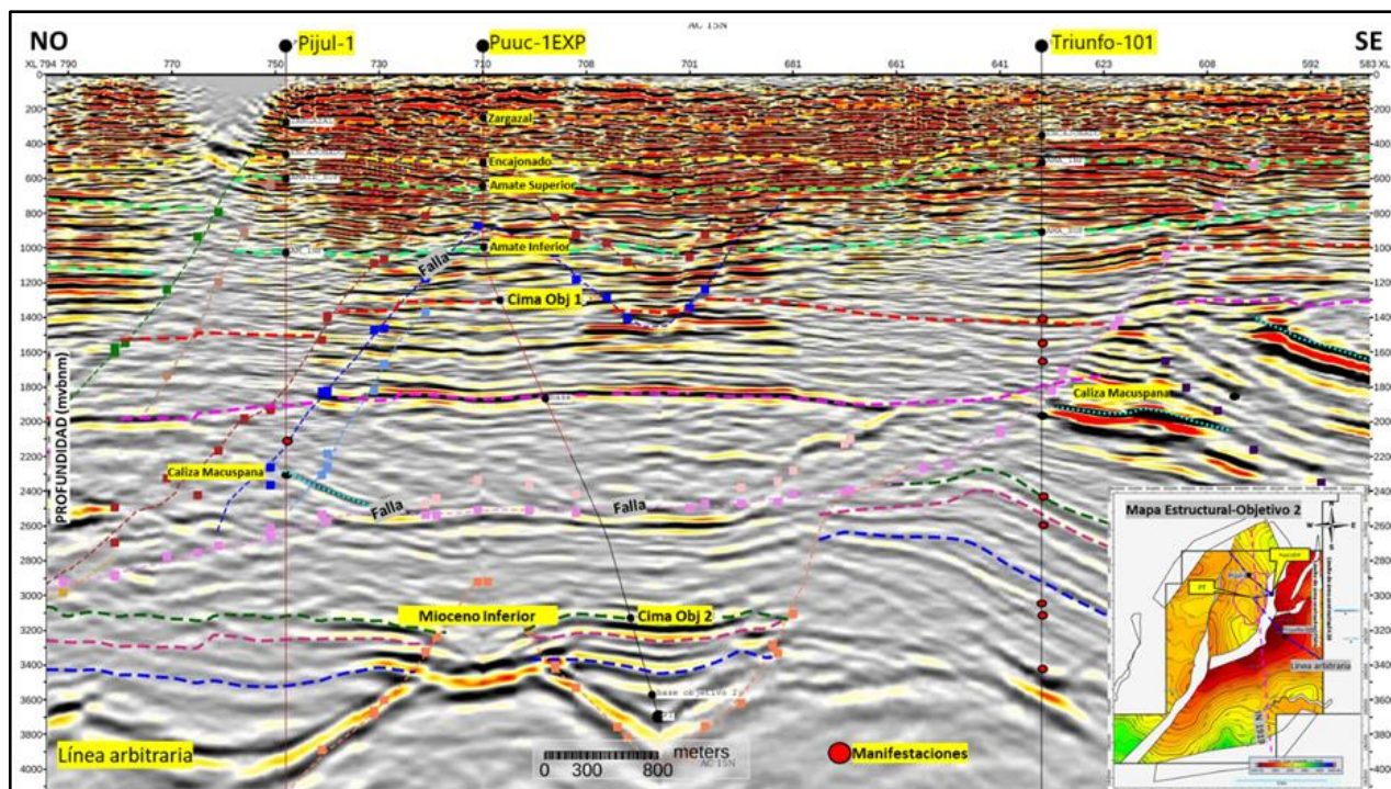
Figura 12. Sección sísmica NO-SE sobre el pozo Puuc-1EXP y los pozos de correlación Pijul-1 y Triunfo-101.
