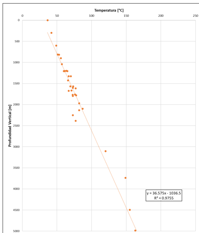
Figura 5. Estimación del gradiente geotérmico de la localización.
