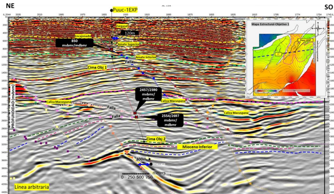
Figura 15. Sección sísmica NE-SO en la que se muestran las fallas circundantes a la localización.
