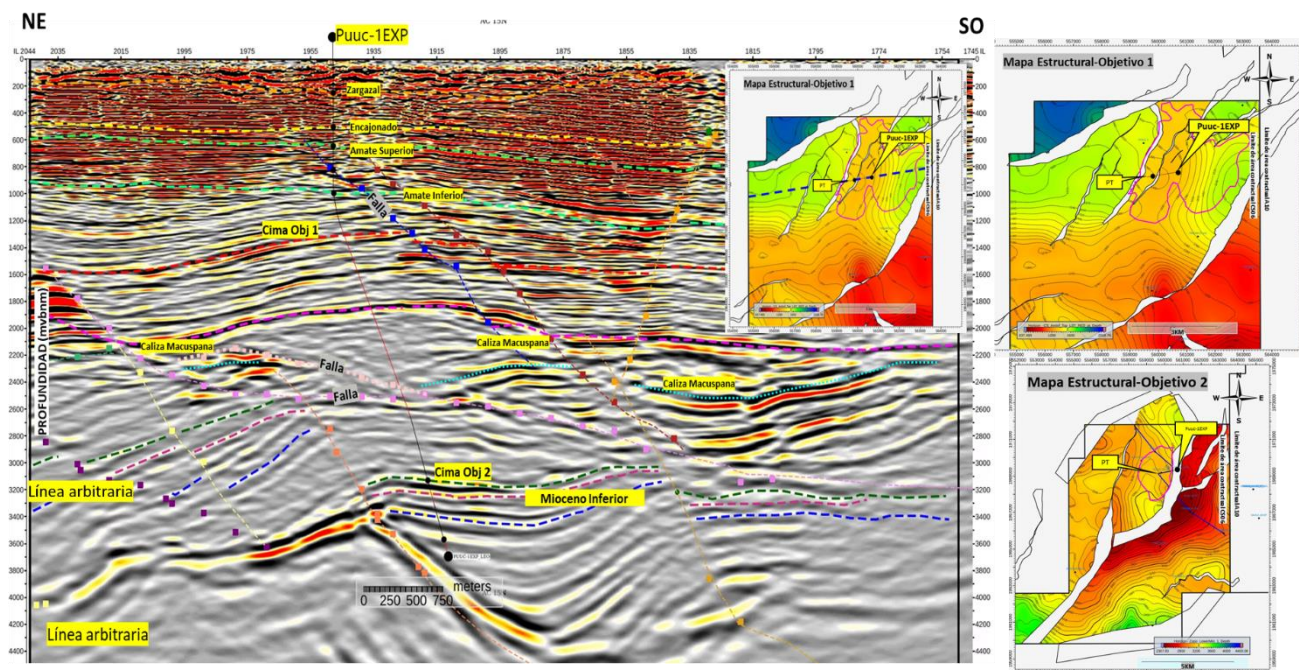
Figura 7. Ubicación estructural del pozo Pucc-1EXP y los rasgos sísmicos de las Formaciones Amate Inferior y el Mioceno Inferior.
