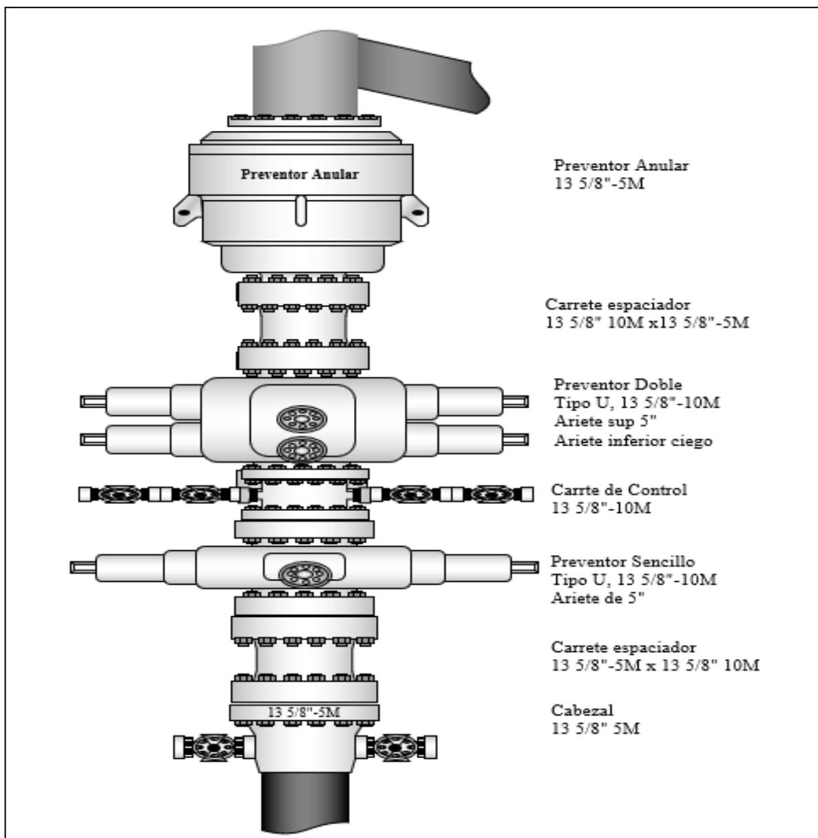
Figura 26. Arreglo 13 \frac{5}{8} " 10M y preventor anular 13 \frac{5}{8} " 5M, para la etapa 12 \frac{1}{4} ".
