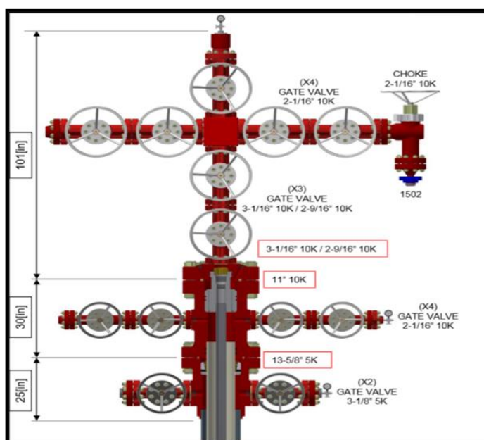
Figura 28. Arreglo preliminar de cabezales y árbol para el proyecto pozo Pucc-1EXP.
