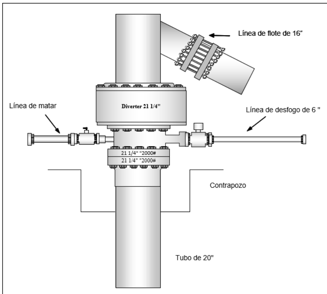
Figura 25. Arreglo del carrete de control y desviador de flujo 21 1/4" x 2M psi para Etapa 17 1/2" - Pucc-1 EXP
