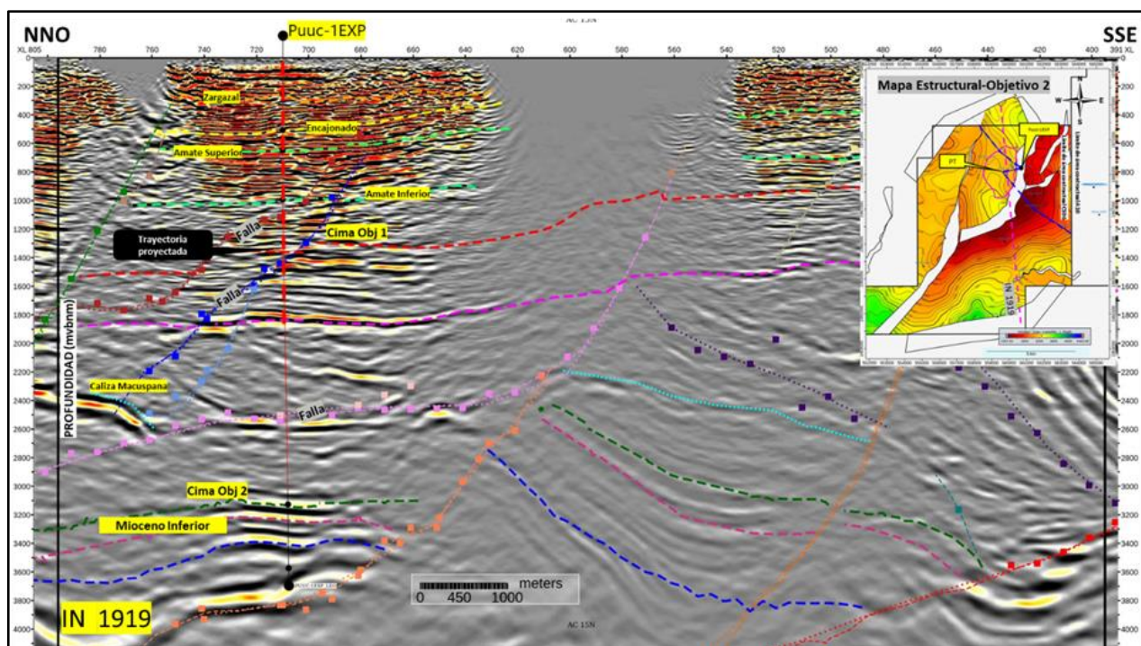
Figura 11. Sección sísmica NNO-SSE sobre el Objetivo 2 en el pozo Puuc-1EXP. Trayectoria sobre Objetivo 1 está proyectada.
