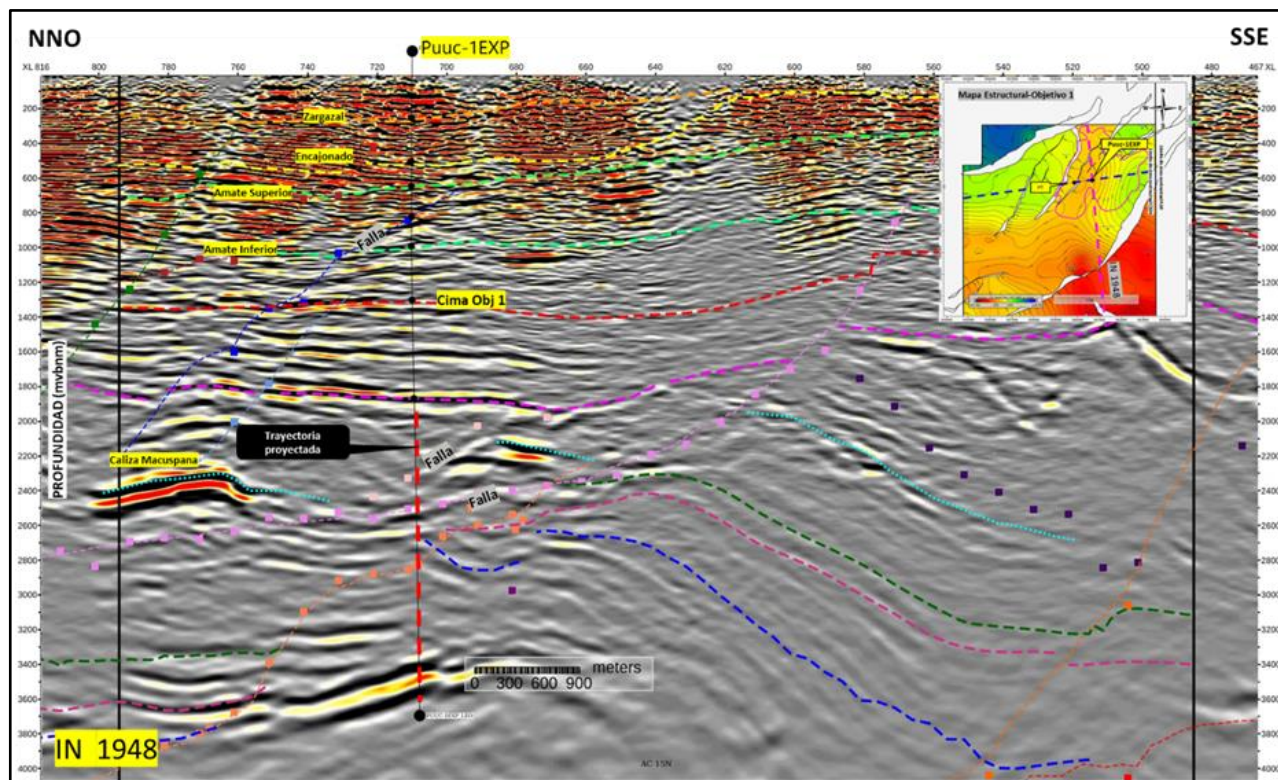
Figura 10. Sección sísmica NNO-SSE sobre el Objetivo 1 en el pozo Puuc-1EXP. Trayectoria sobre Objetivo 2 está proyectada.
