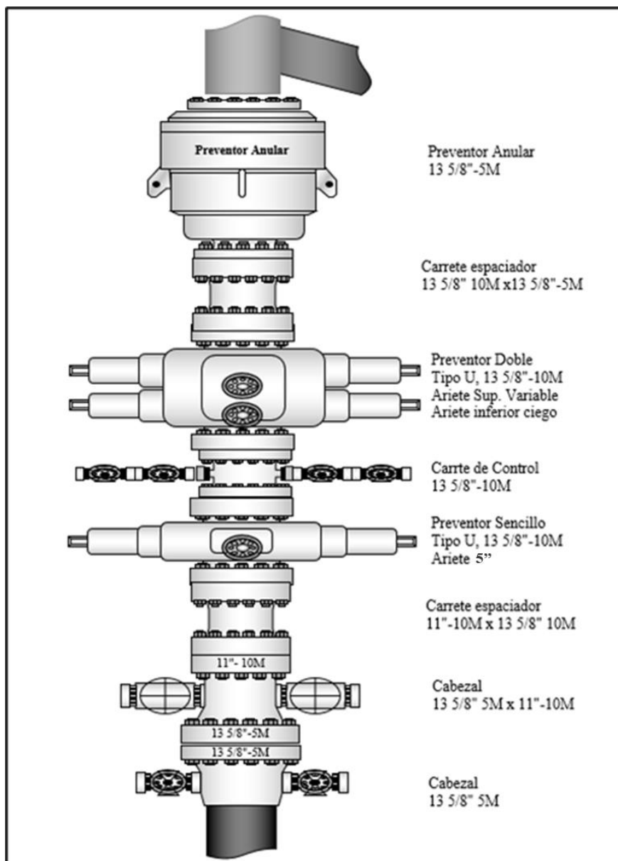
Figura 19. Arreglo de Preventor Esférico de 13 5/8" 5M con Ariete Superior Variable y Ariete Inferior Ciego, Carrete de Control de 13 5/8" 10M con Salidas Laterales de 3 1/16" 10M y Válvula Mecánica de 3 1/8", Brida de 3 1/16", Preventor Sencillo de 13 5/8" 10M y Cabezal 11" 10M para la Etapa 8 1/2"
