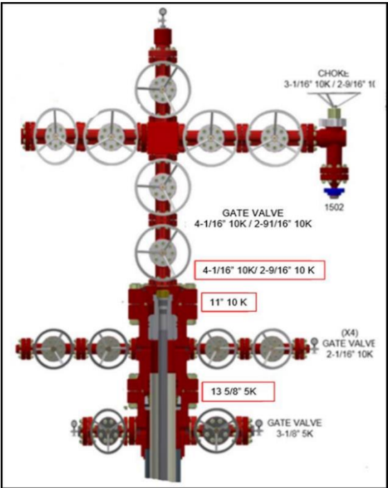
Figura 20. Arreglo de cabezales y árbol para el proyecto pozo Pípila-45DES.
