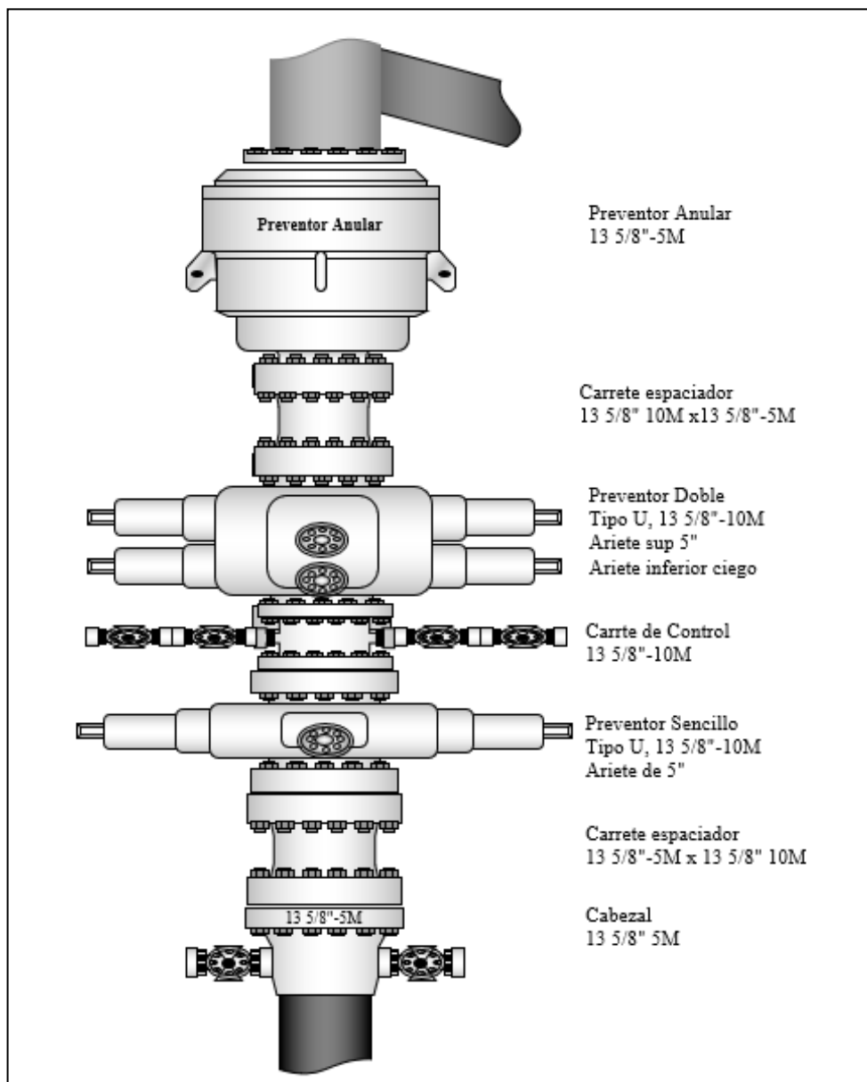
Figura 18. Arreglo 13 5/8" 10M y Preventor Anular de 13 5/8" 5M, para la etapa de 12 1/4"
