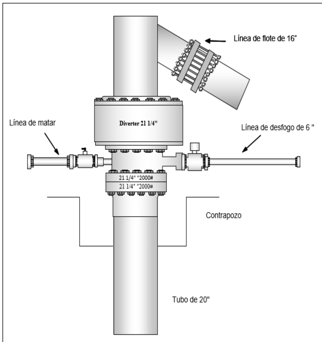
Figura 17. Arreglo del carrete de control y desviador de flujo 21 ¼" x 2M, etapa de 17 ½"
