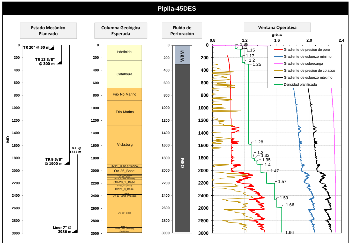
Figura 7. Estado mecánico propuesto para el pozo Pípila-45DES.
