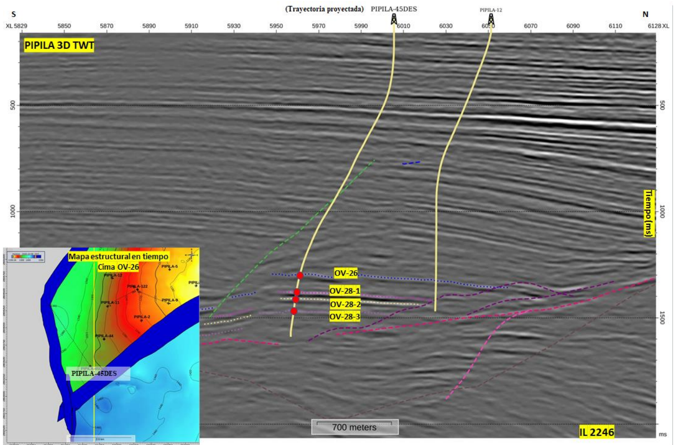
Figura 5. Sección sísmica en tiempo IL 2246. Se muestran los rasgos estructurales principales indicándose los objetivos de interés. Se observa la trayectoria desviada con el fin de penetrar los objetivos en áreas donde se predicen mejores condiciones de reservorios. Las fallas principales se muestran con líneas discontinuas y los horizontes con líneas punteadas. Debido a que la trayectoria del pozo mostrada está proyectada, se parece que se va a cruzar una falla (color verde discontinua) pero no la va a encontrar.
