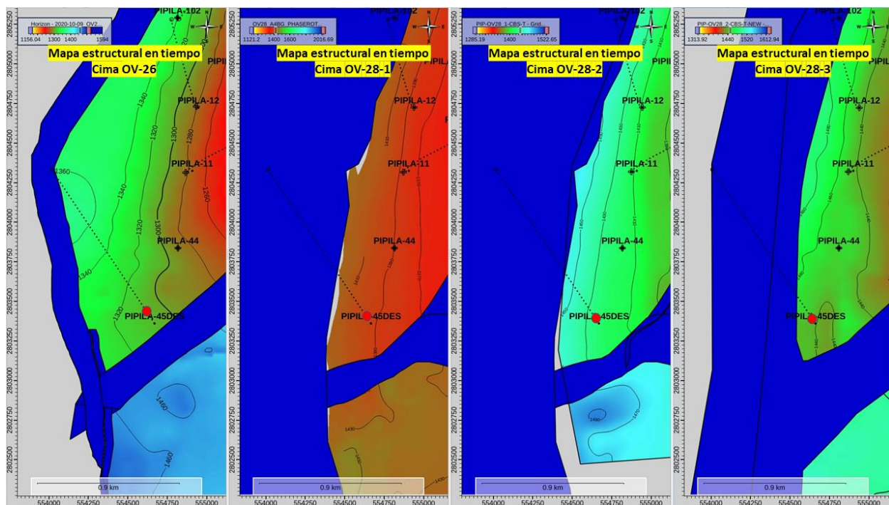
Figura 2. Mapas estructurales en tiempo de los principales objetivos del Campo Pípila, donde se muestra la localización Pípila-45DES. Para la interpretación y el mapeo del área se usó una versión PSTM del estudio sísmico PIPILA 3D. Los círculos rojos corresponden a la ubicación donde la trayectoria del pozo penetra al objetivo.
