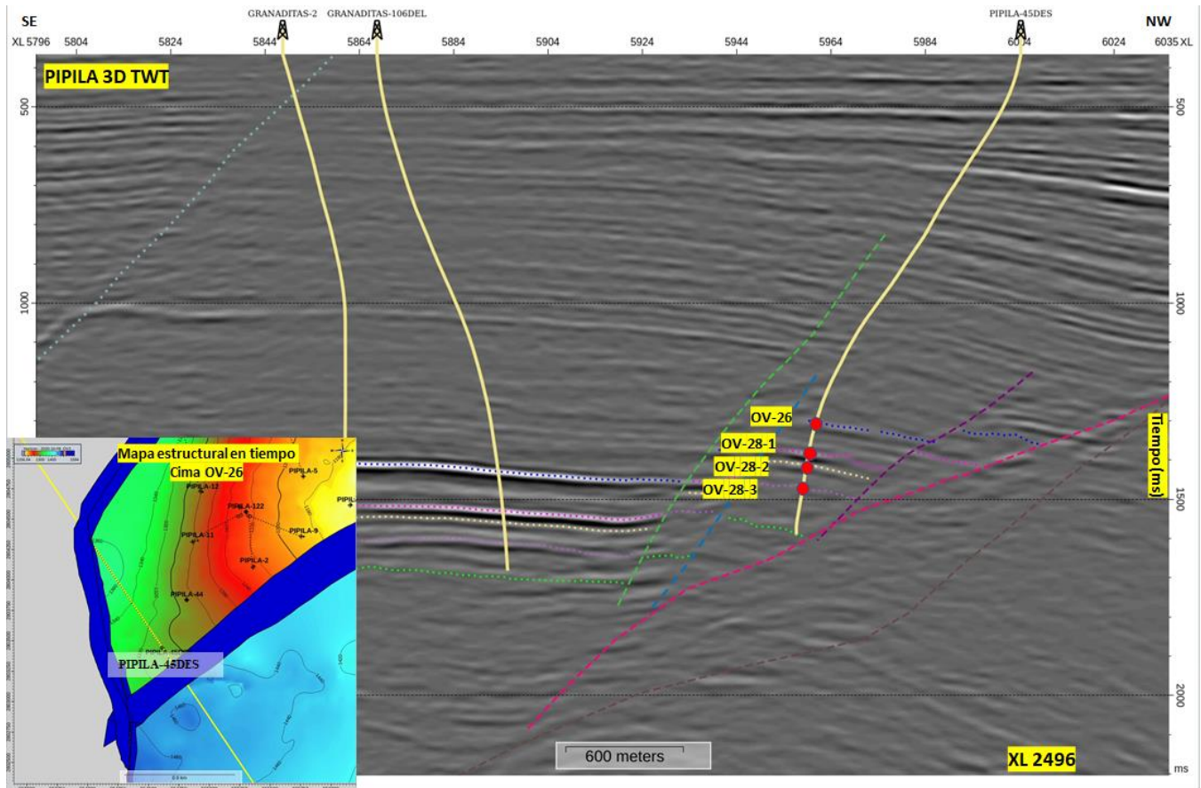
Figura 6. Sección sísmica arbitraria en tiempo sobre la trayectoria del pozo. Se puede visualizar la trayectoria verdadera en la sísmica, en la cual se observa que a pesar de la cercanía a las fallas no las cruza.
