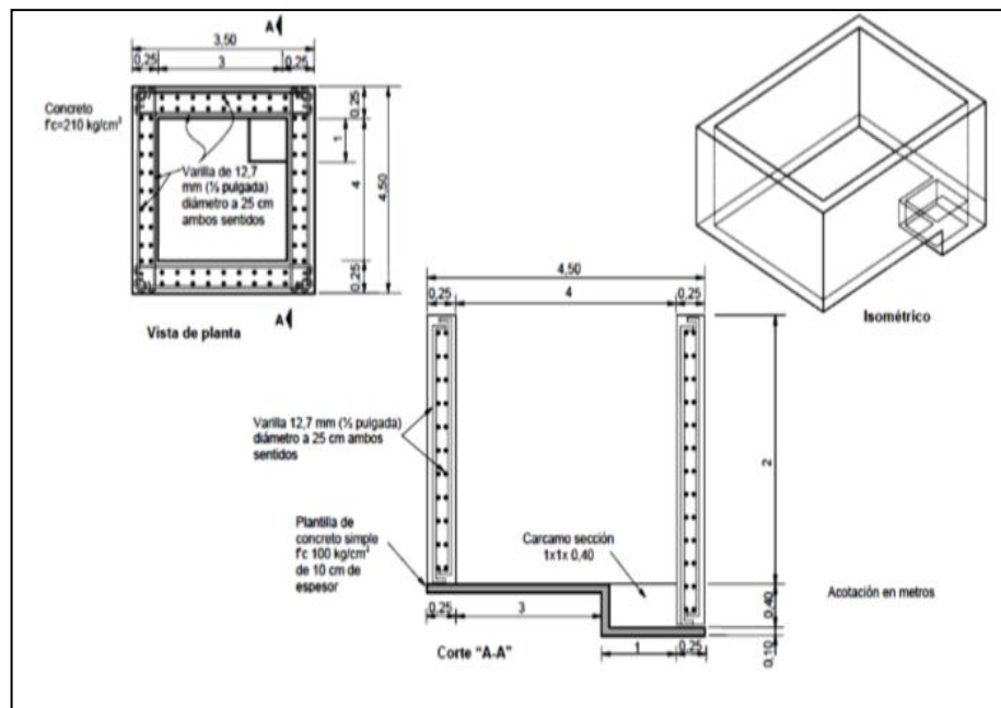
Figura 15. Diseño del contra pozo.
