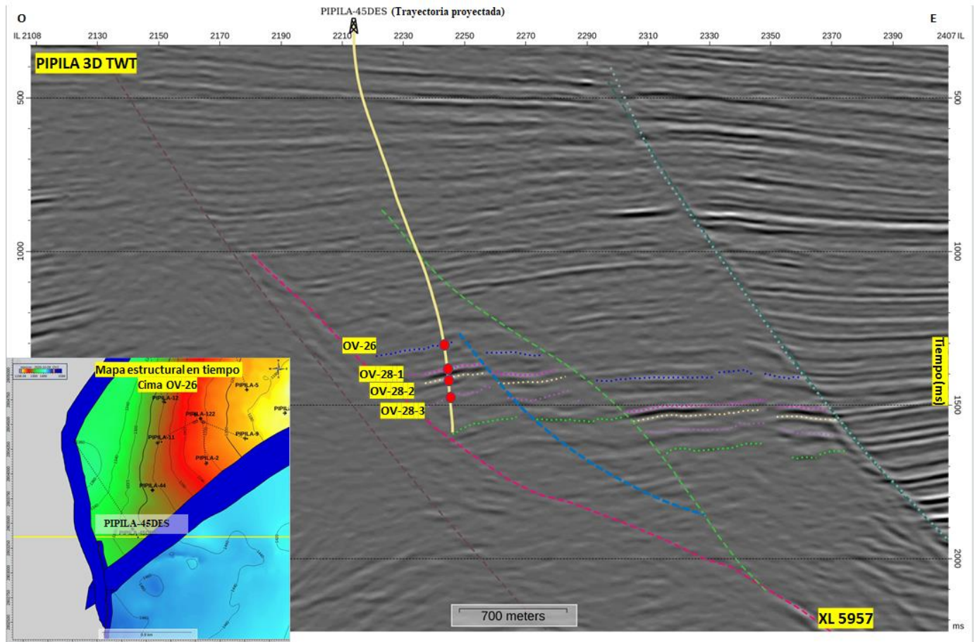
Figura 4. Sección sísmica en tiempo XL 5957. Se muestran los rasgos estructurales principales indicándose los objetivos de interés. Se observa la trayectoria desviada con el fin de penetrar los objetivos en áreas donde se predicen mejores condiciones de reservorios. Las fallas principales se muestran con líneas discontinuas y los horizontes con líneas punteadas. Debido a que la trayectoria del pozo mostrada está proyectada, se parece que se va a cruzar una falla (color verde discontinua) pero no la va a encontrar.
