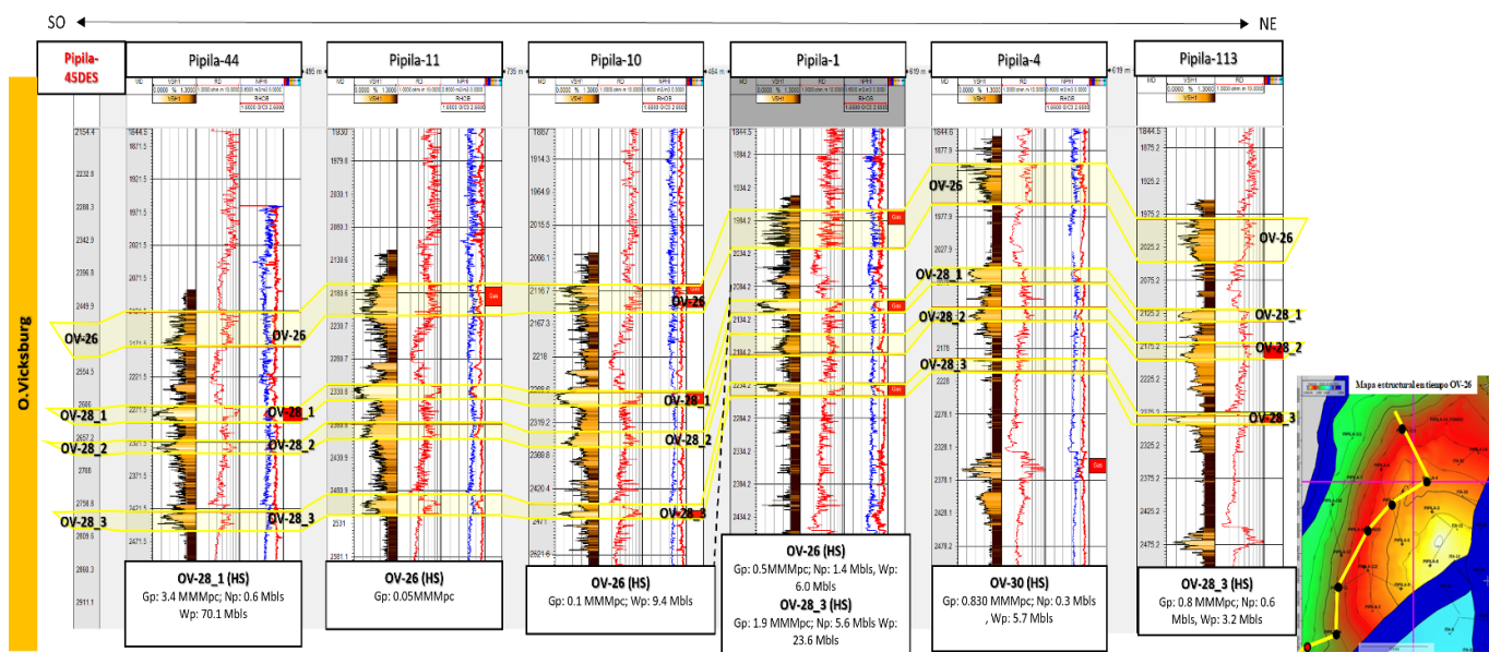
Figura 3. Correlación estructural a nivel de Oligoceno Vicksburg, en la cual se observa la continuidad de las principales arenas de interés entre la localización Pípila-45DES y los pozos vecinos.
