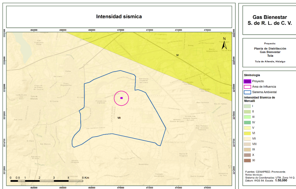
Figura IV.17. Intensidad sísmica.
