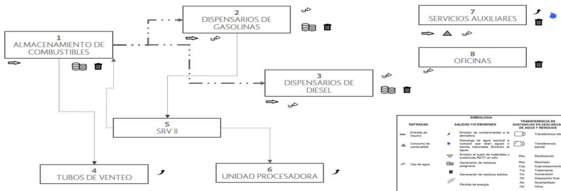
DIAGRAMA DE FUNCIONAMIENTO (GENERAL)
