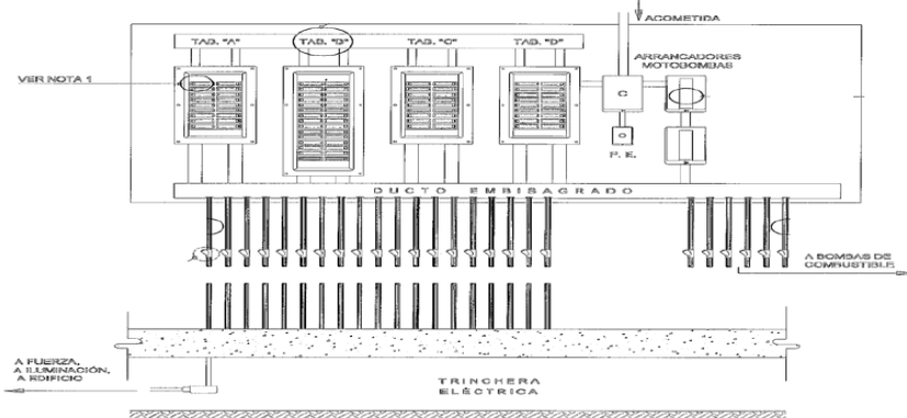
IMAGEN 8. TABLERO ELÉCTRICO
