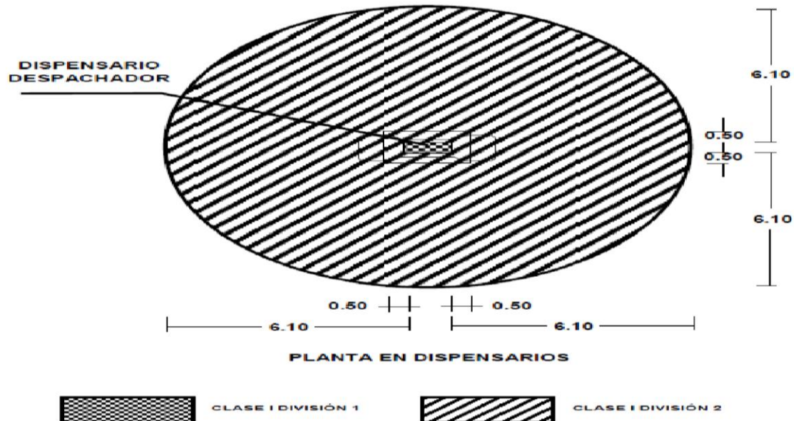
IMAGEN 6. CLASIFICACIÓN DE ÁREA PELIGROSA DISPENSARIO
