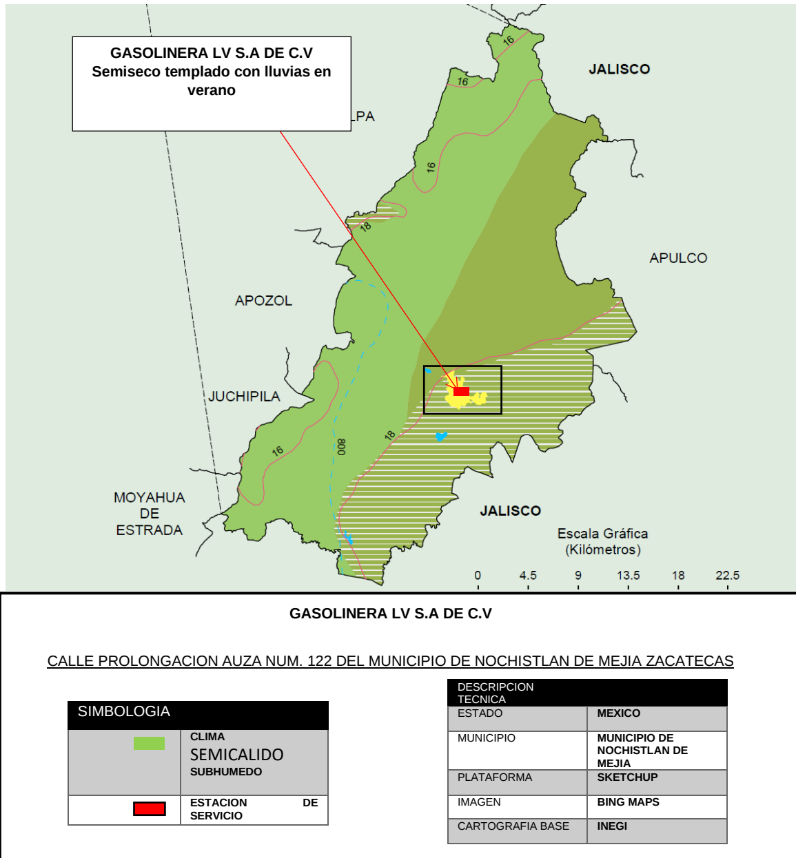
Imagen 16. Clima de que incide en el área del proyecto
