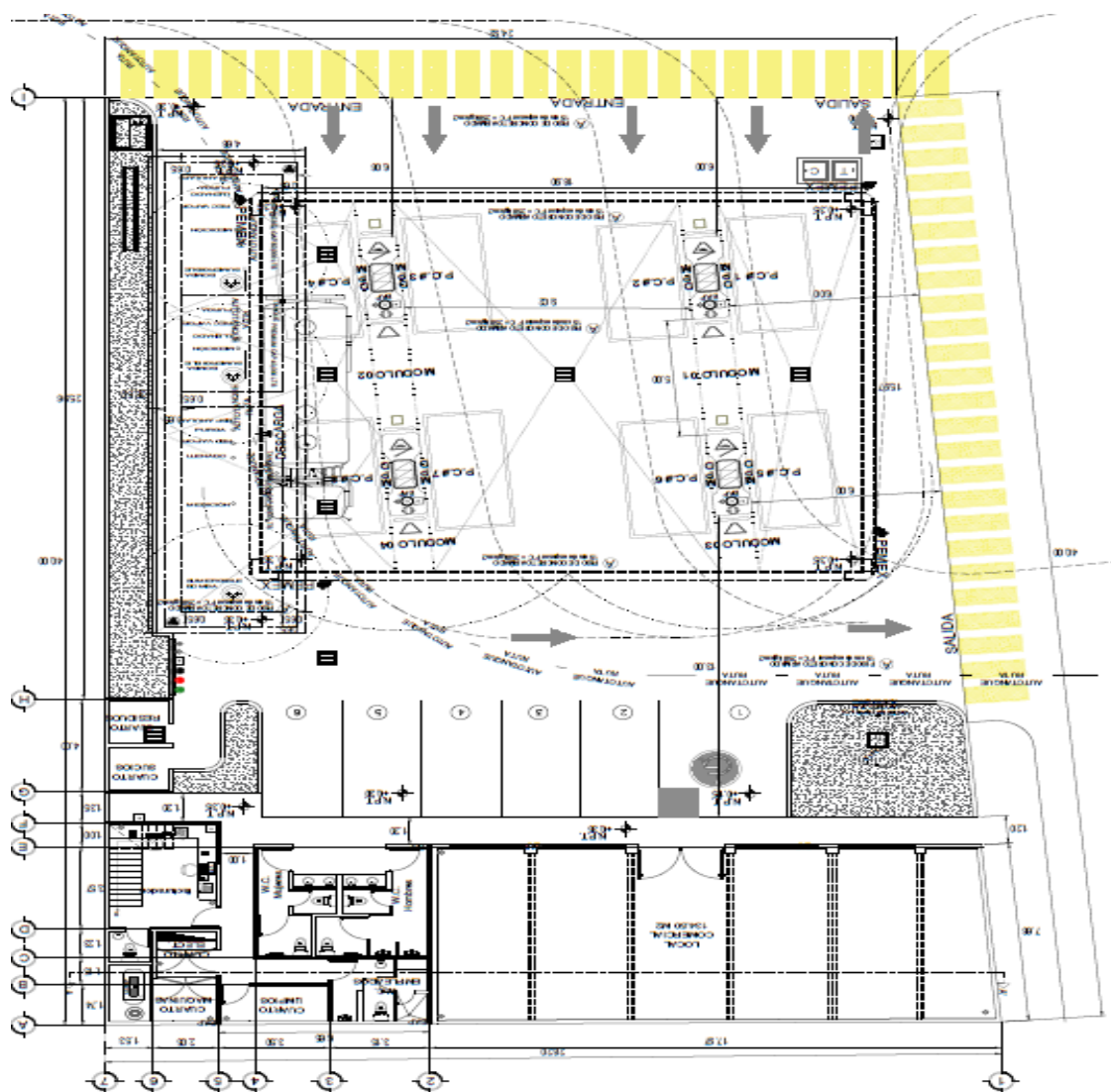
Imagen 11. Plano de Conjunto de GASOLINERA LV S.A DE C.V
