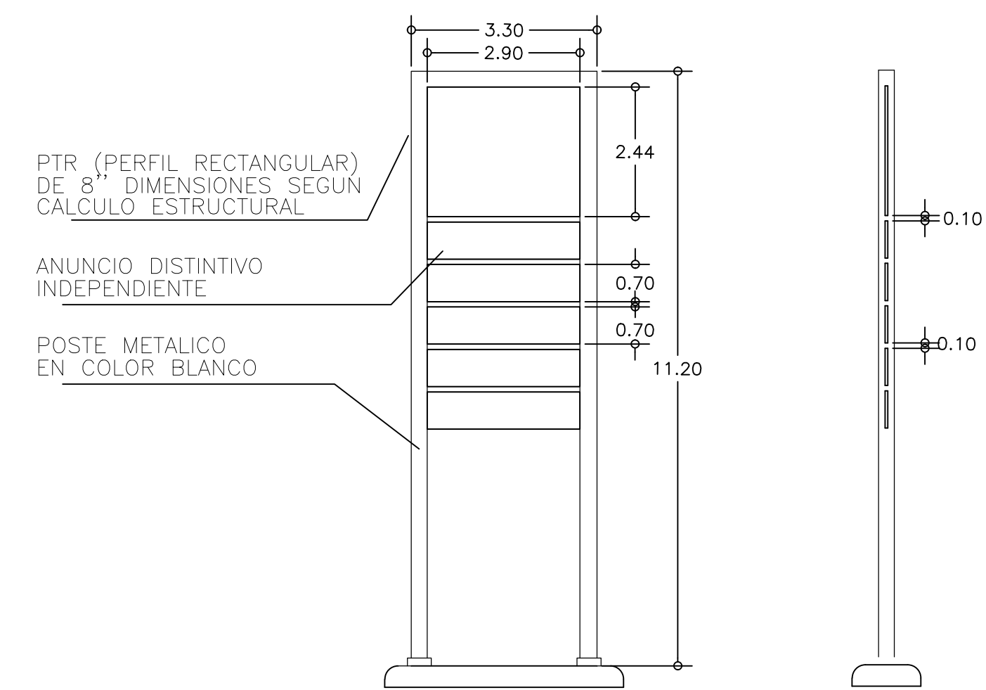
02 ANUNCIO INSTITUCIONAL ESC 1:100
