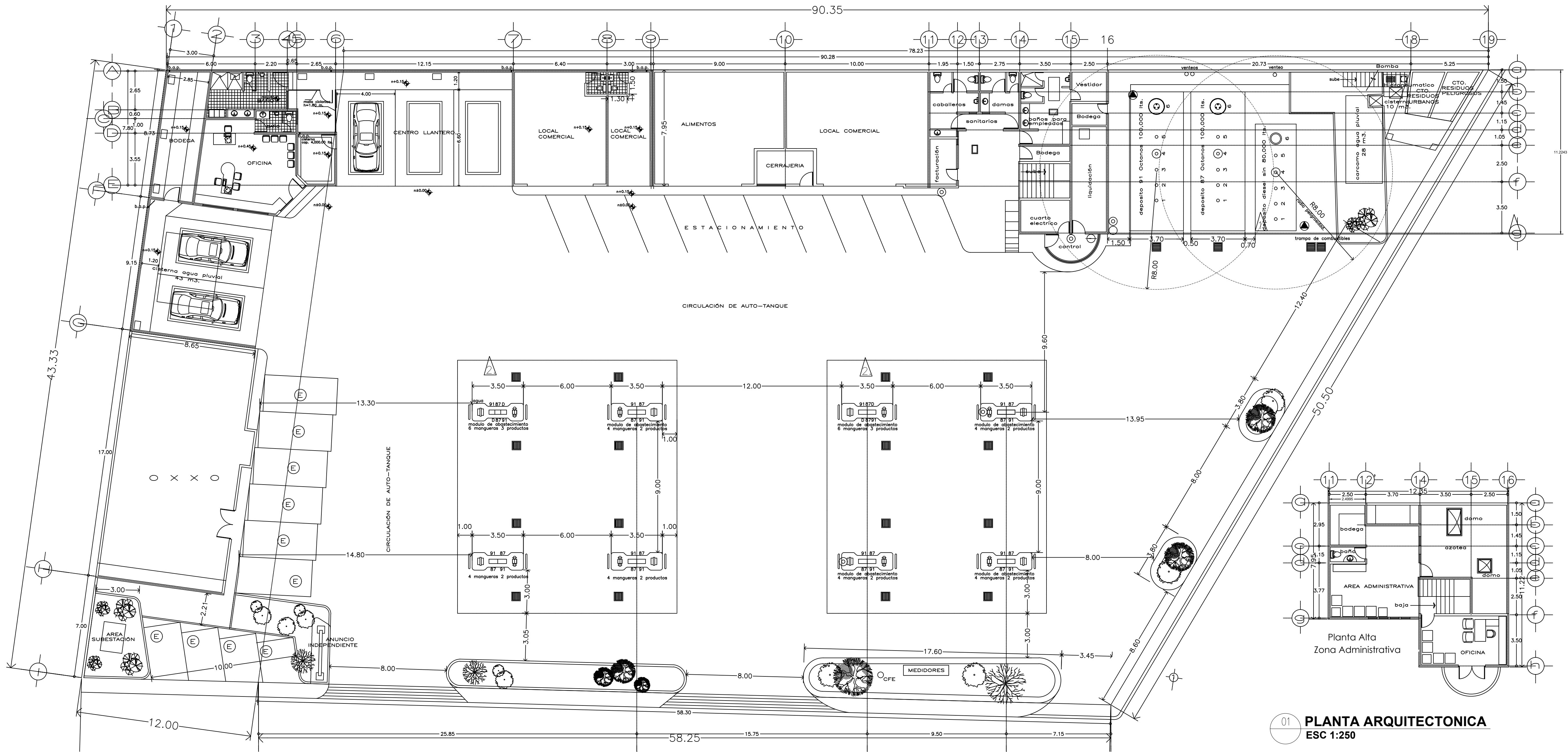
01 PLANTA ARQUITECTONICA ESC 1:250
