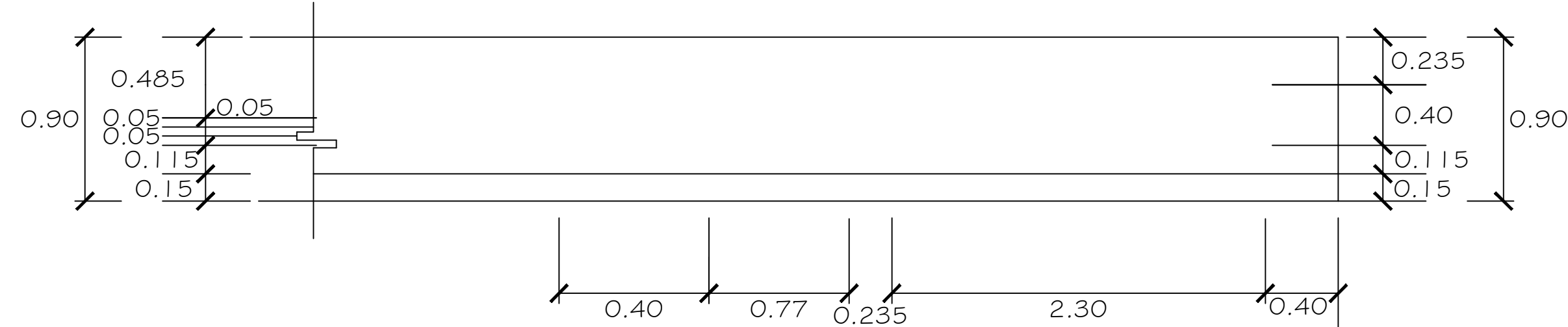
03 DETALLE FALDON PERIMETRAL SIN ESCALA
