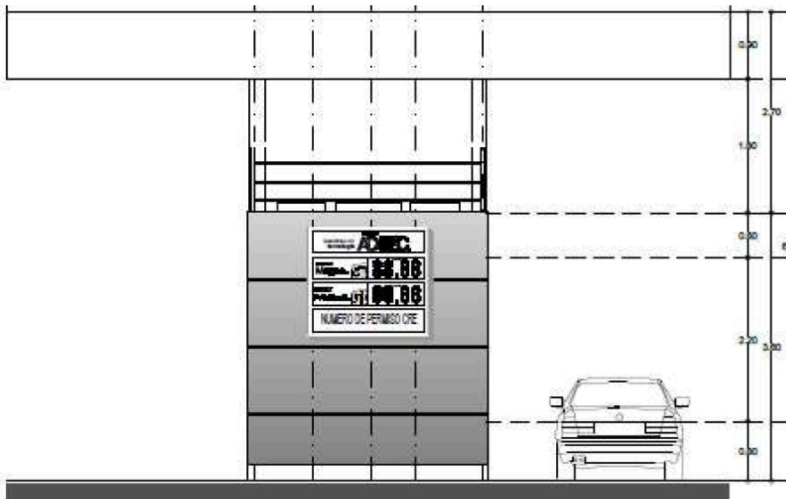
FACHADA LATERAL ESTACION DE SERVICIO ALZADO ESCALA 1:50
