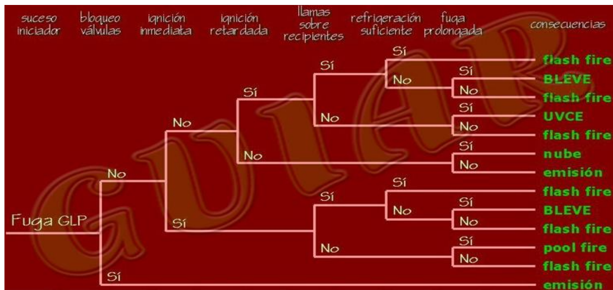
Figura 23. Árbol de sucesos para fuga de gas L.P. en zona próxima a los tanques de almacenamiento.
