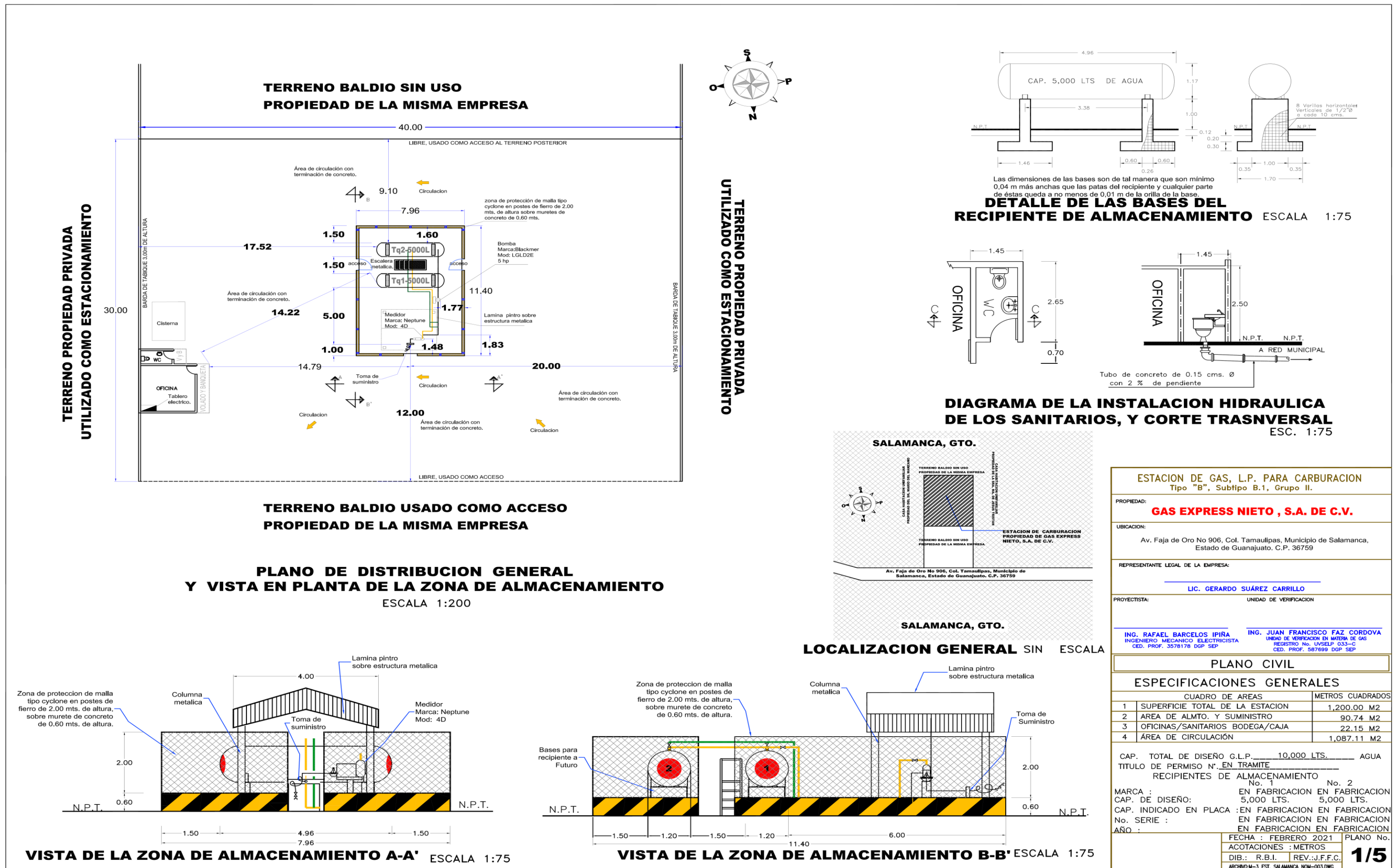
Figura 4. Distribución de áreas dentro del predio (arreglo general de la estación de carburación).
