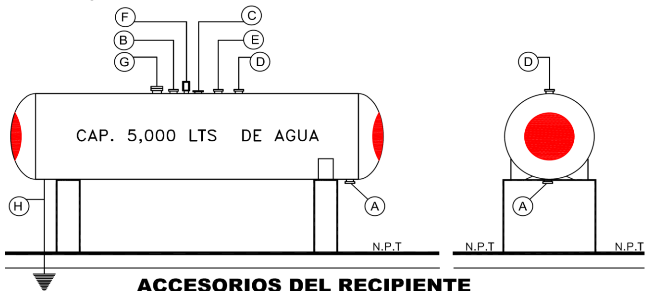
Figura 12. Instrumental de seguridad de los tanques de almacenamiento.
