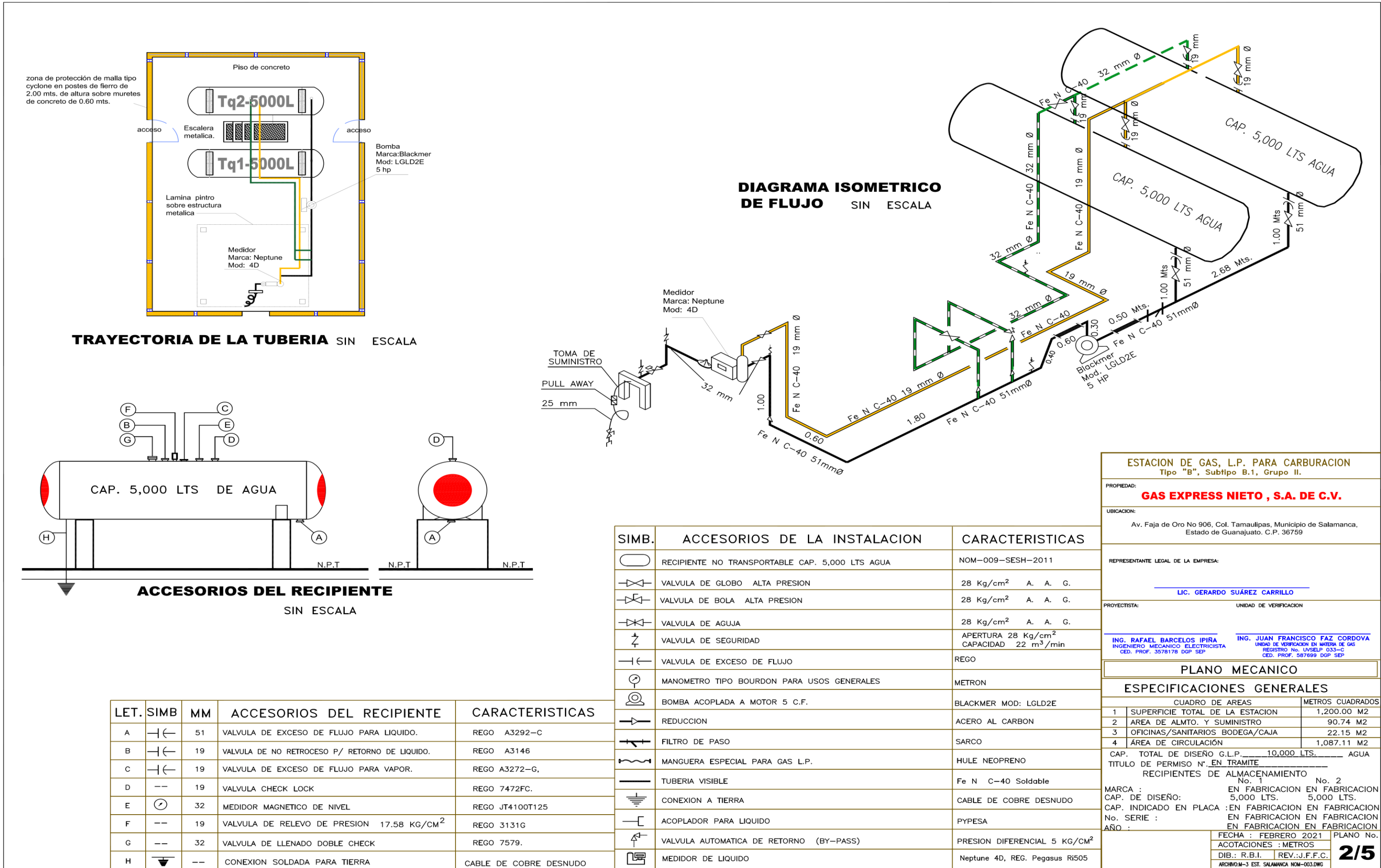
Figura 4_b. Plano mecánico sin escala con detalles de los tanques de almacenamiento y equipamiento de la estación proyectada..
