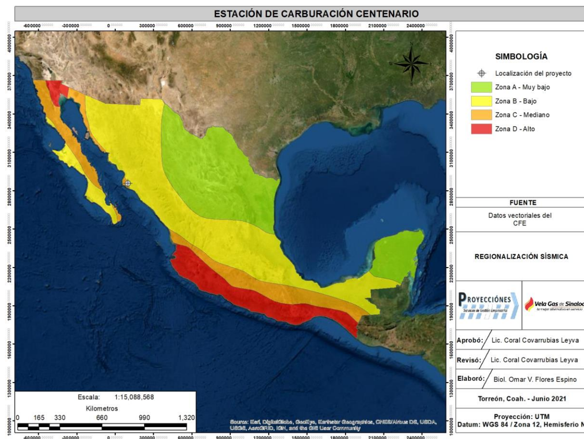
Figura 4. Regionalización sísmica.
