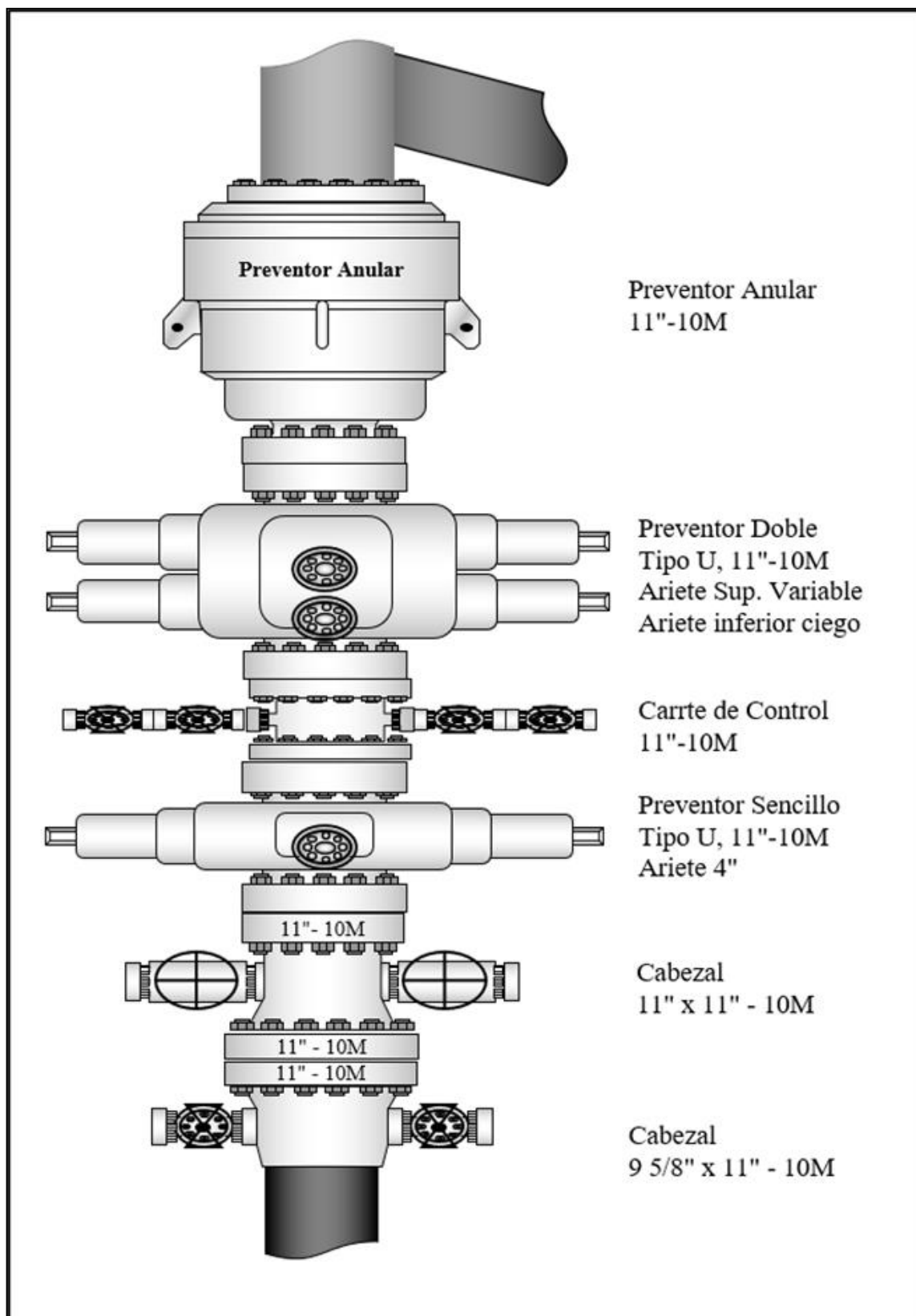
Figura 27. Arreglo 11" 10M y Preventor Anular de 11" 10M, para la etapa de 8 1/2".
