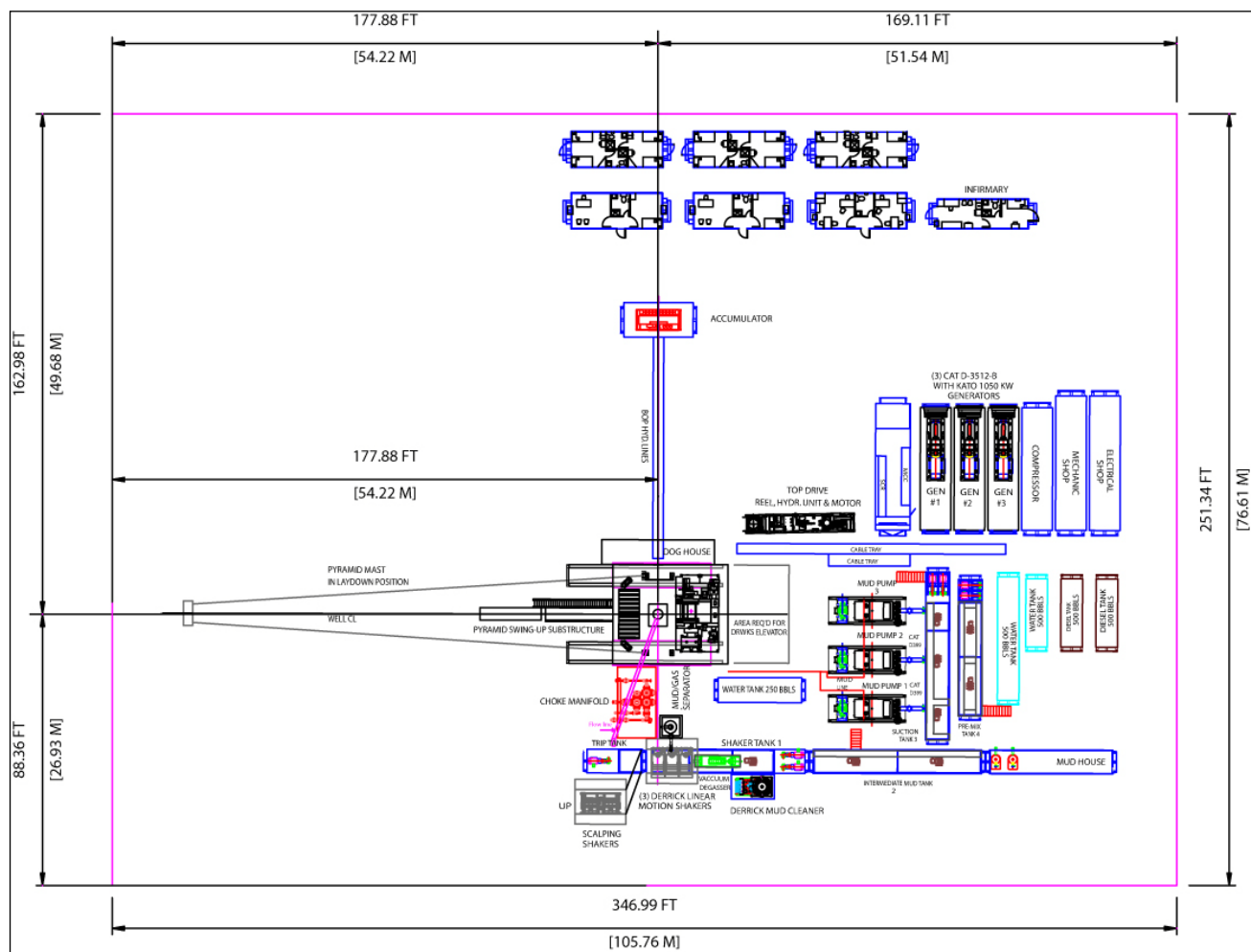
Figura 25. Diseño del arreglo de un equipo de perforación de 2.000 HP
