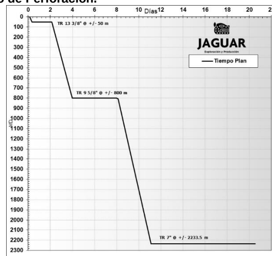
Gráfica de tiempo vs. Profundidad
