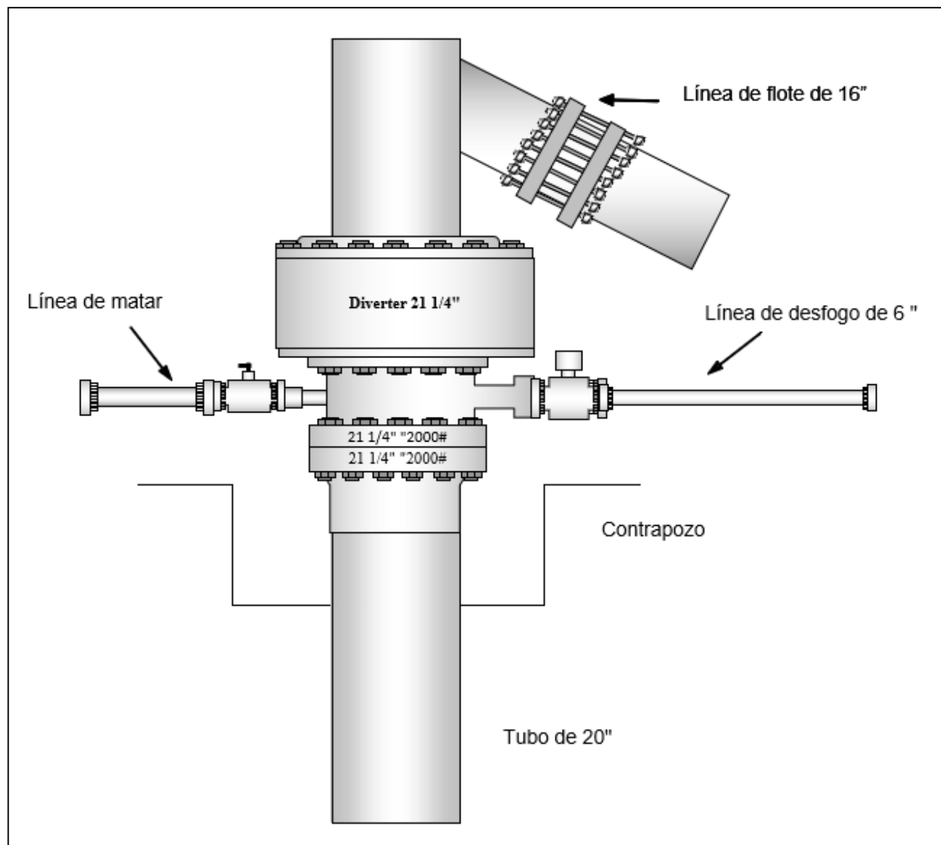
Figura 26. Arreglo del carrete de control y desviador de flujo 21 1/4" x 2M psi para Etapa 12 1/4". Nota: Se cuenta con la brida de 13 5/8" 5M con cuello soldable, así como con la brida adaptadora de 13 5/8" 5M x 21 1/4" 2M.
