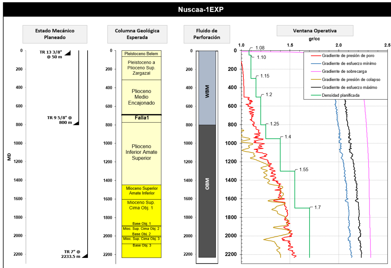
Figura 2. Estado mecánico del pozo
