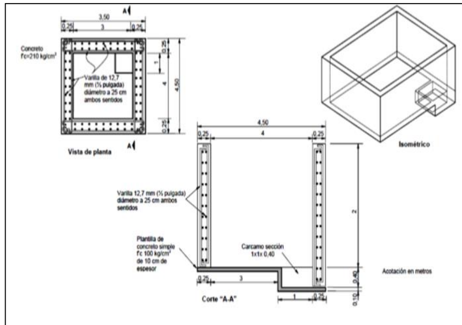
Figura 24. Diseño del contra pozo.
