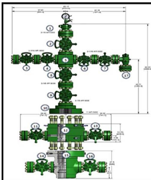
Figura 28. Arreglo preliminar de cabezales y árbol para el proyecto pozo Kinkan-1EXP.
