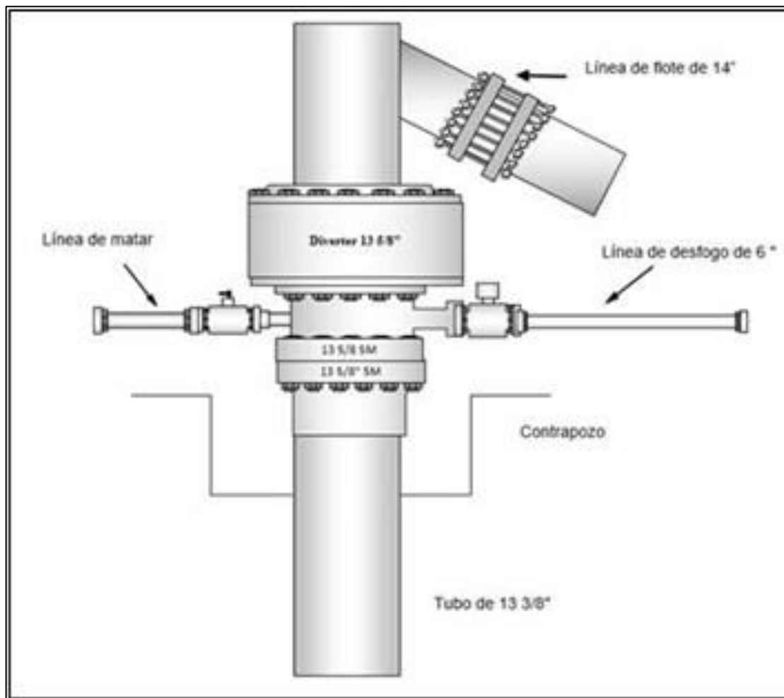
Figura 26. Arreglo de desviador de flujo 13 5/8" para Etapa 12 1/4"
