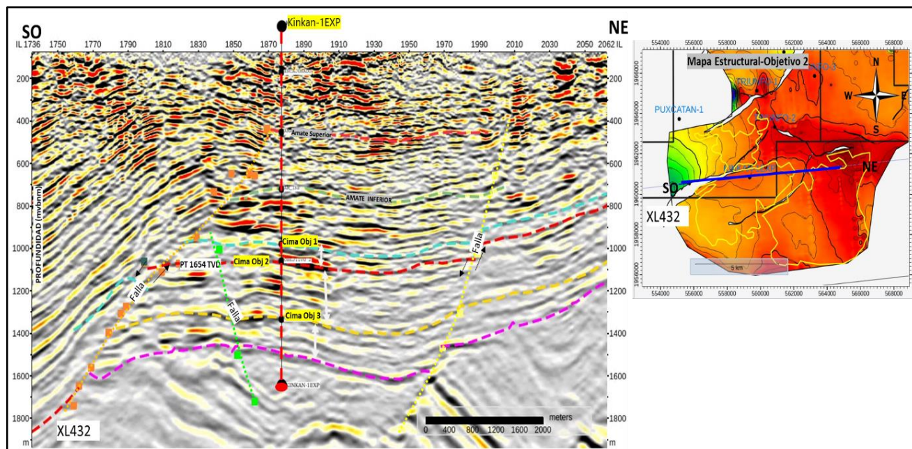
Figura 12. Sección sísmica OSO-ENE sobre el pozo Kinkan-1EXP y mapa estructural de la cima del objetivo 2.
