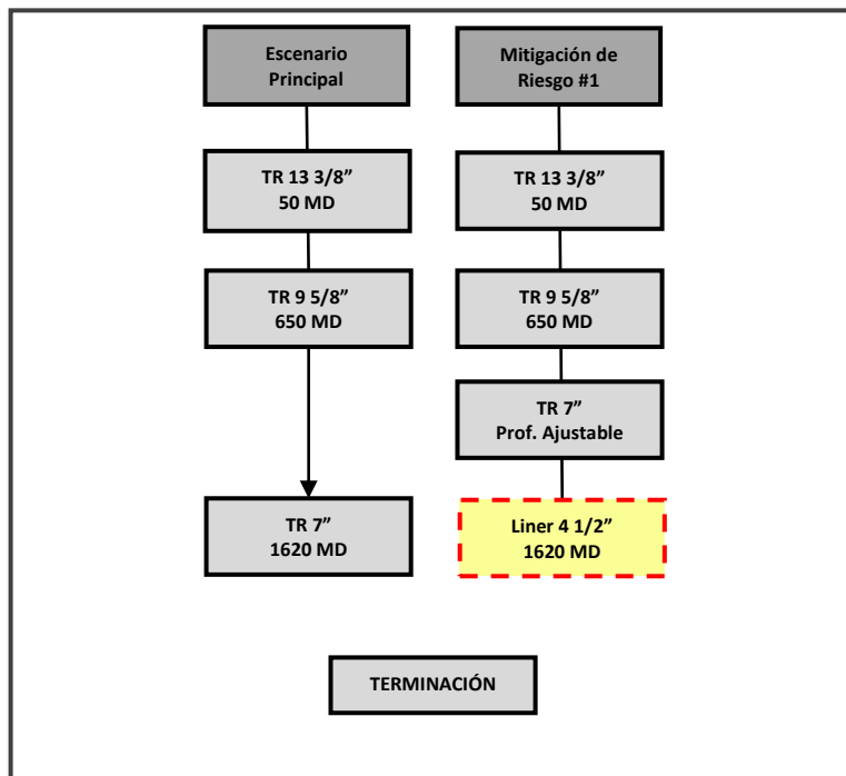
Figura 3. Escenarios de Mitigación de Riesgos para el proyecto pozo Kinkan-1EXP.
