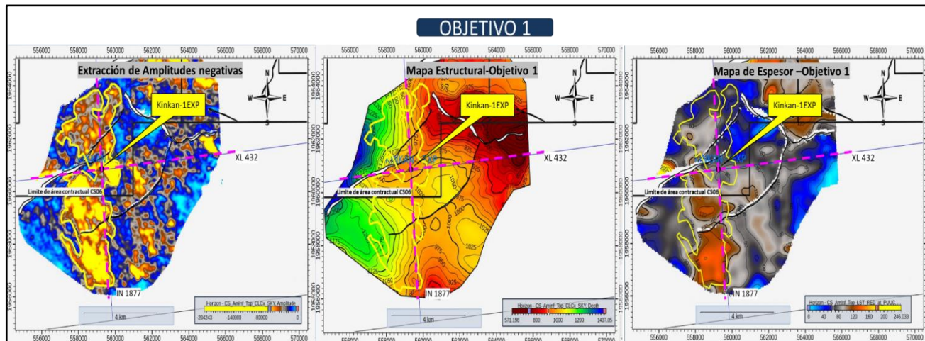
Figura 14. Mapas de atributo sísmico, estructural y espesor de objetivo 1.
