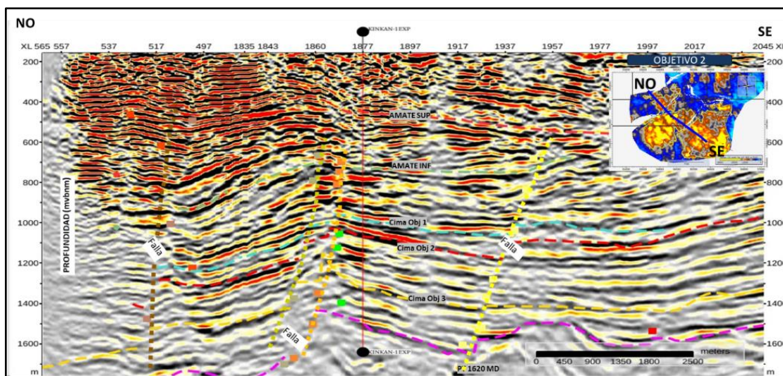
Figura 10. Sección sísmica arbitraria NO-SE sobre el pozo Kinkan-1EXP, mapa de extracción de suma de amplitudes negativas en objetivo 2.
