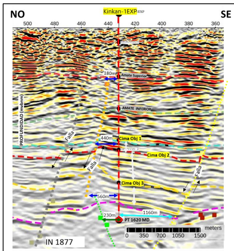
Figura 17. Sección sísmica NO-SE en la que se muestran las fallas circundantes a la localización.
