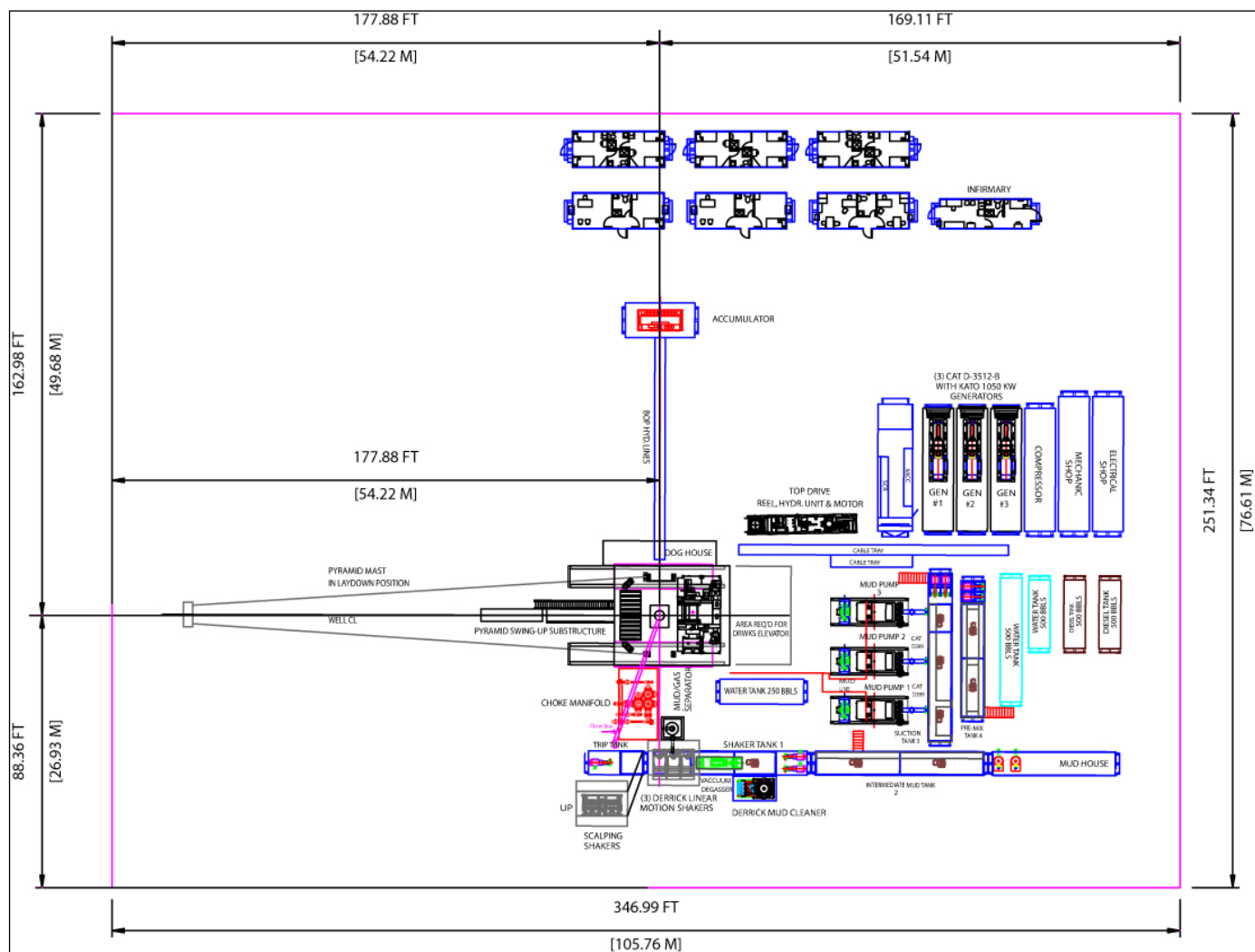
Figura 25. Diseño del arreglo de un equipo de perforación de 2.000 HP
