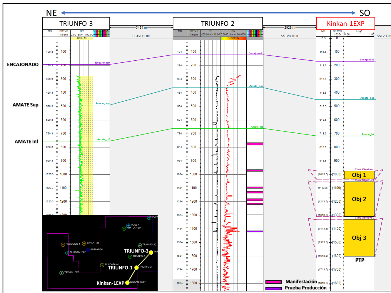
Figura 8. Correlación estructural de localización Kinkan-1EXP y pozos aledaños.
