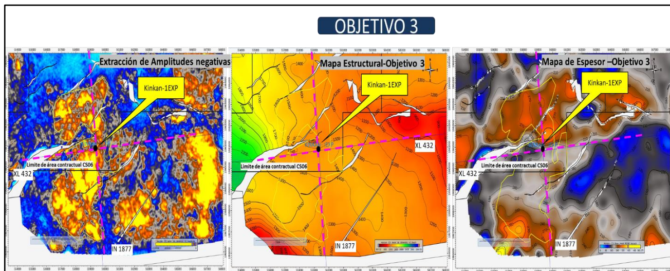
Figura 16. Mapas de atributo sísmico, estructural y espesor de objetivo 3.
