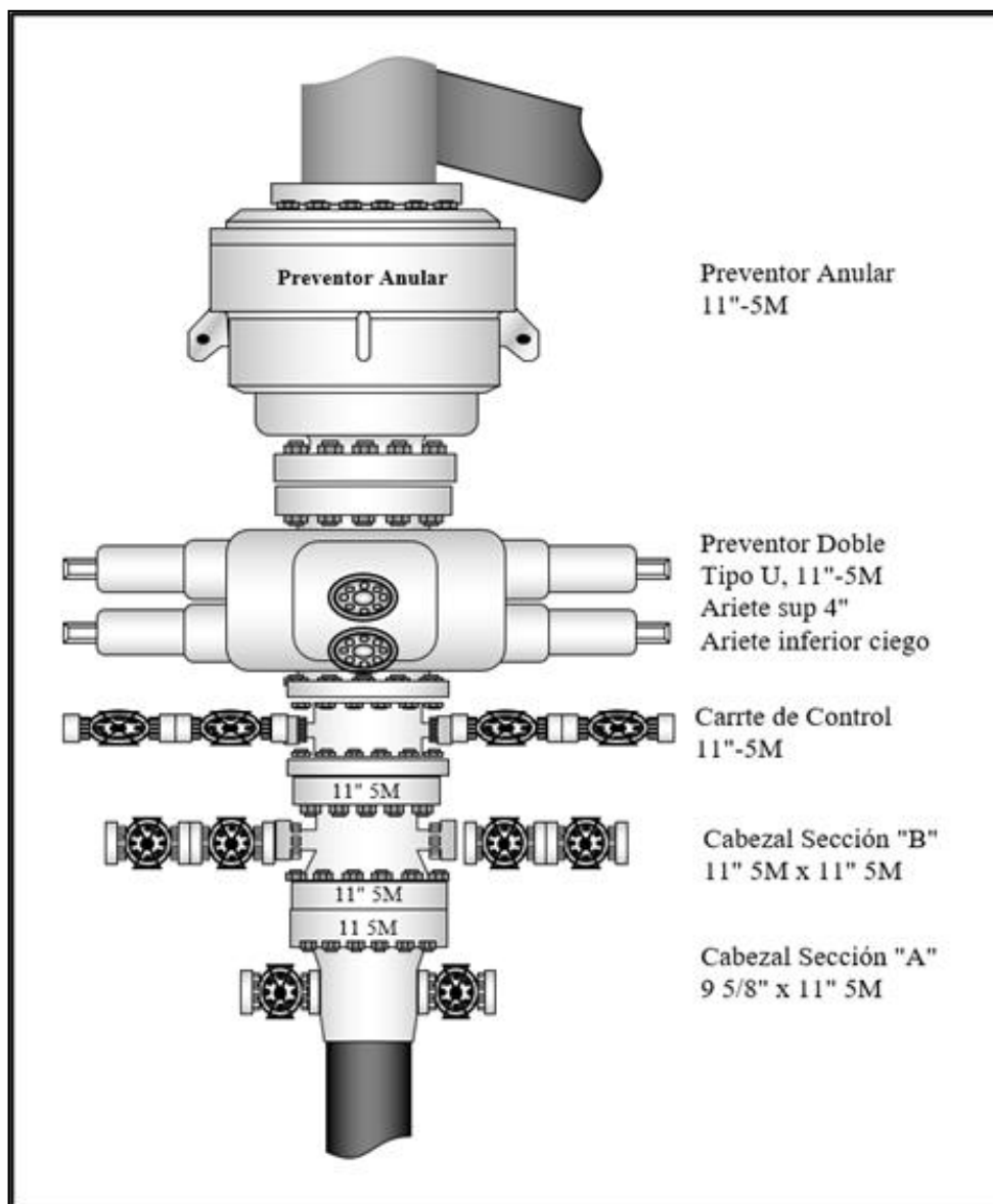
Figura 27. Arreglo 11" 5M y preventor anular de 11" 5M, para la etapa de 8 1/2"
