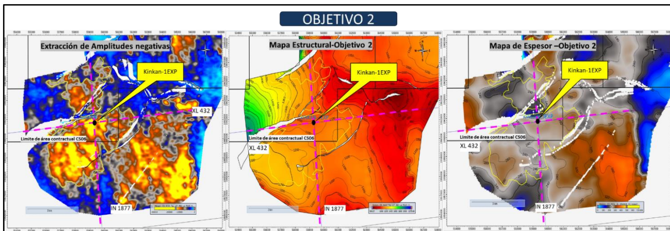
Figura 15. Mapas de atributo sísmico, estructural y espesor de objetivo 2.
