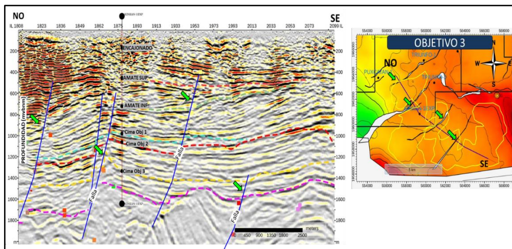
Figura 7. Sección sísmica arbitraria a través del pozo Kinkan-1EXP y mapa estructural de la cima del objetivo 3.
