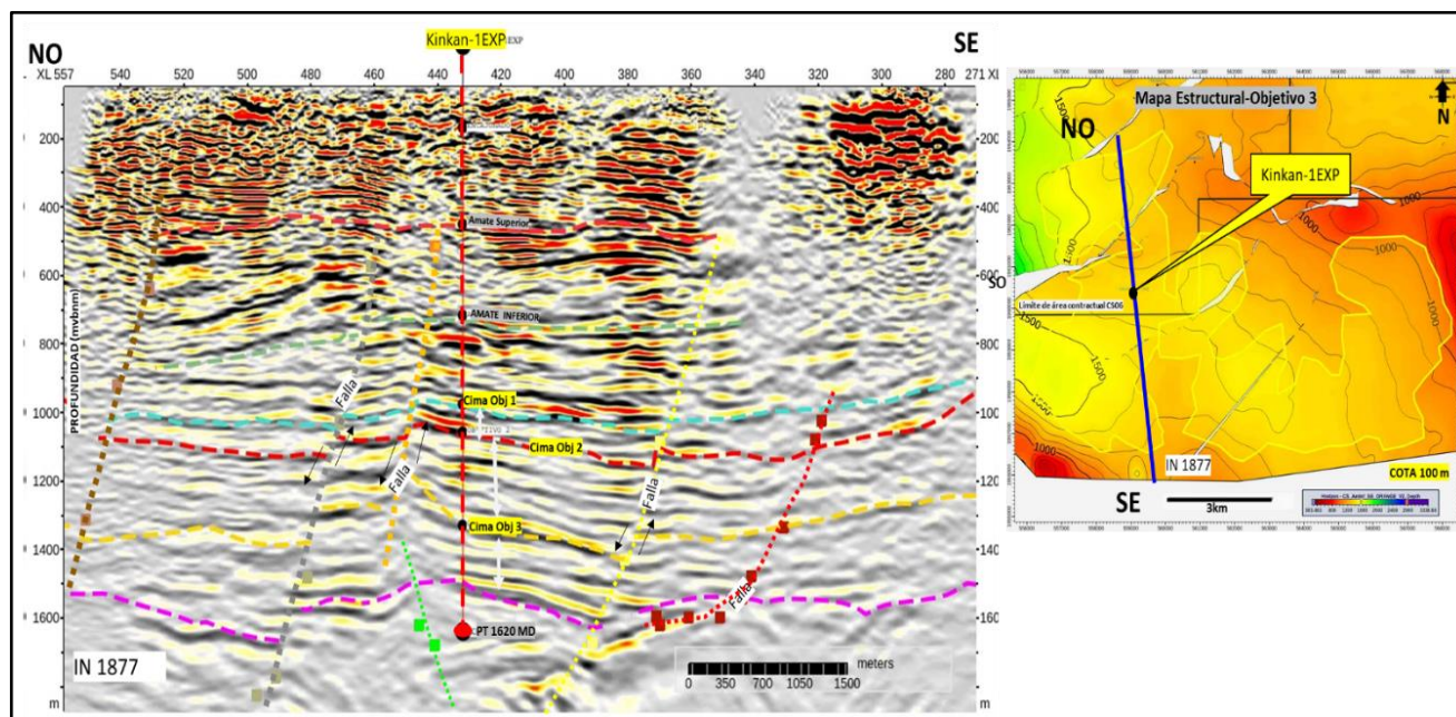
Figura 11. Sección sísmica N-S sobre el pozo Kinkan-1EXP y mapa estructural de la cima del objetivo 3.
