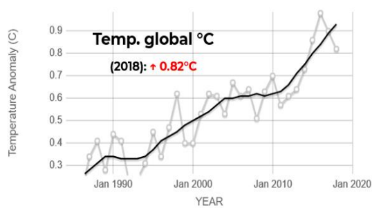
Figura 5. Evolución del incremento de la temperatura global (1990-2020)
