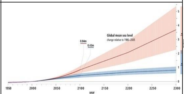
Figura 8. Evolución del incremento del nivel del mar (1950-2300)
