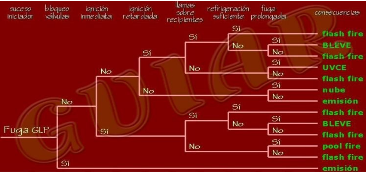
Figura 13. Árbol de sucesos para fuga de gas L.P. en zona próxima al tanque de almacenamiento.
