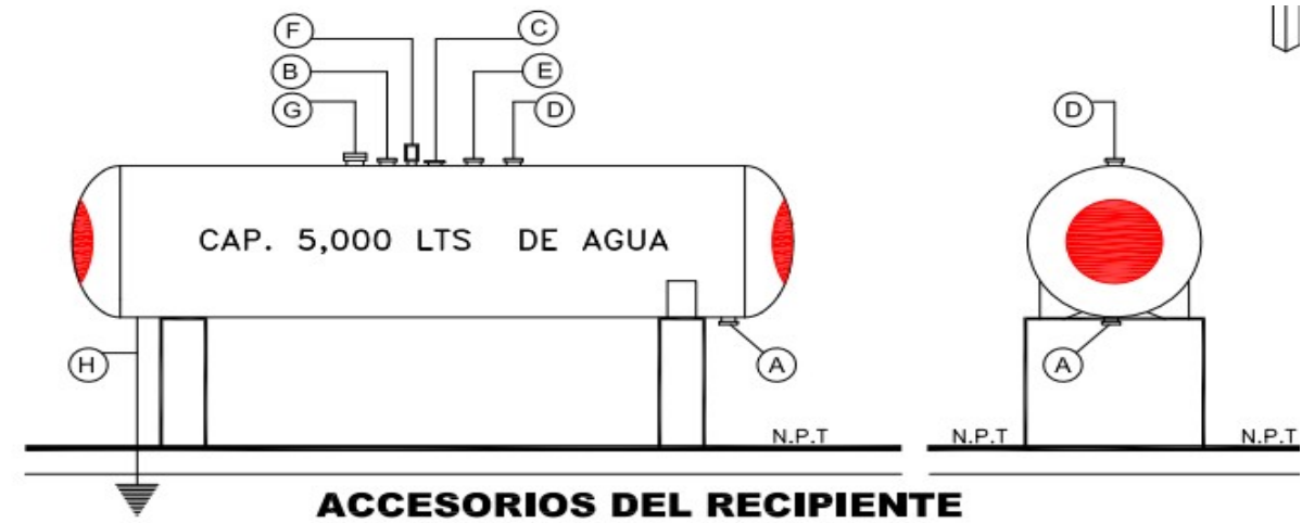
Figura 6. Instrumental de seguridad del tanque de almacenamiento.
