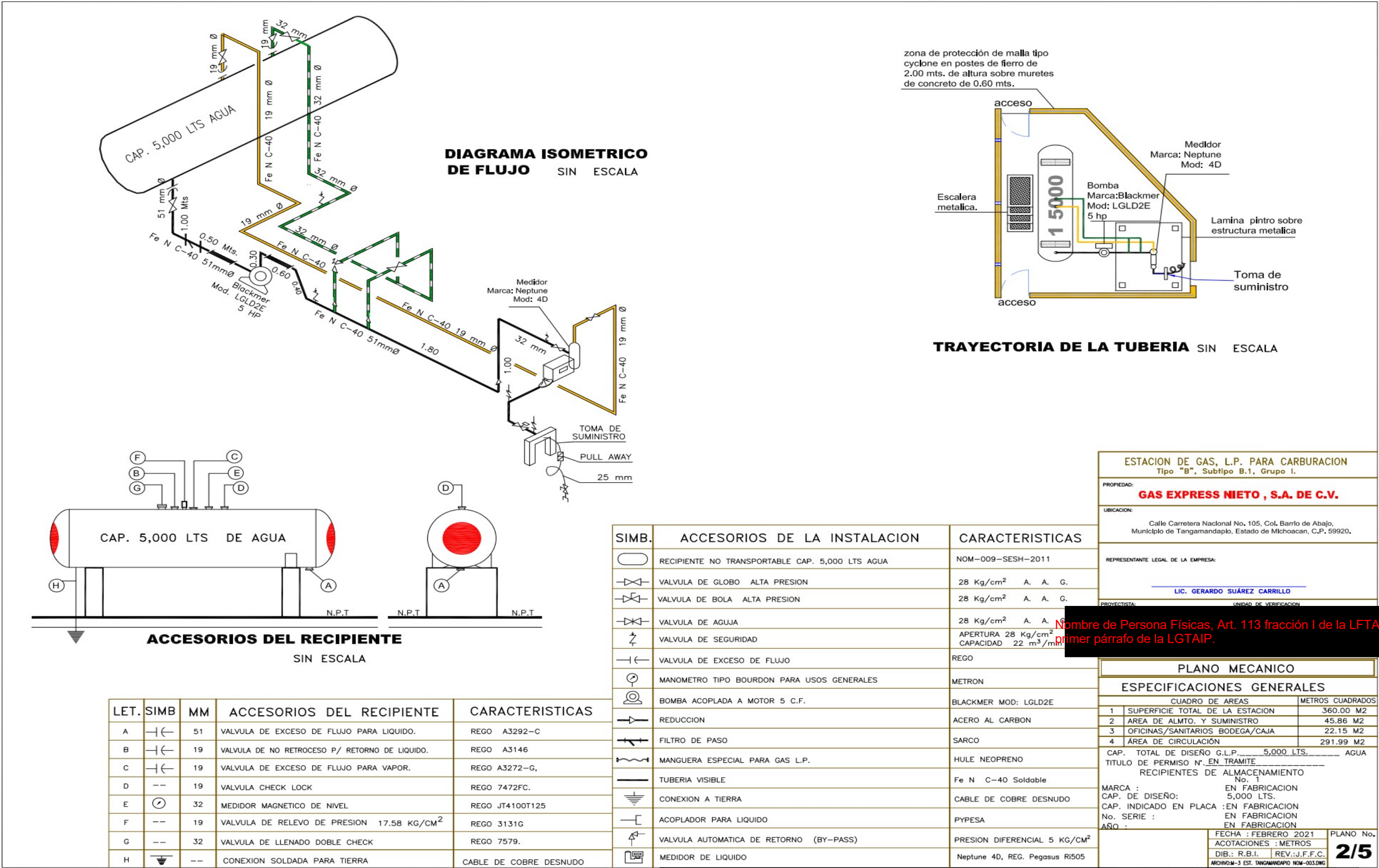
Figura 4_b. Plano mecánico sin escala con detalles del tanque de almacenamiento y equipamiento de la estación proyectada
