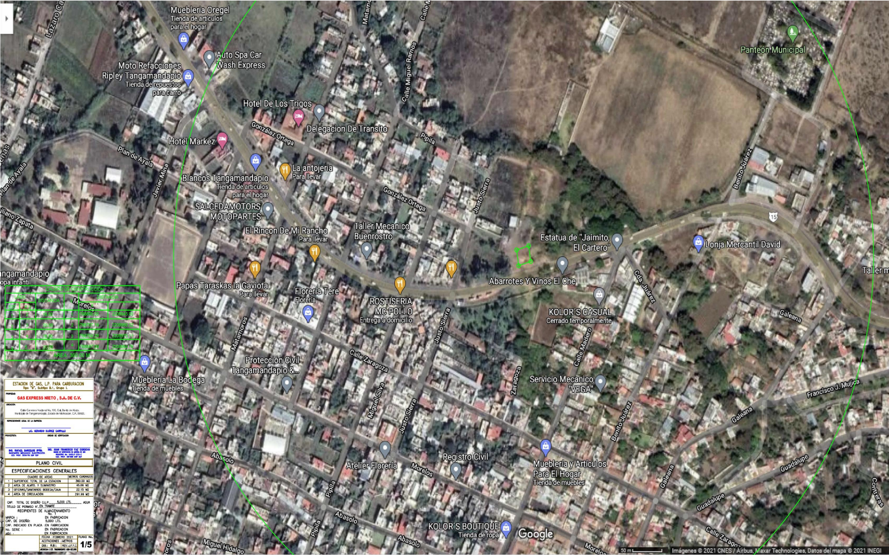
Figura 2.Microlocalización del terreno para la estación de carburación, en una vista de satélite a través de Google maps indicando el tipo de actividades en un radio de 500 metros.
