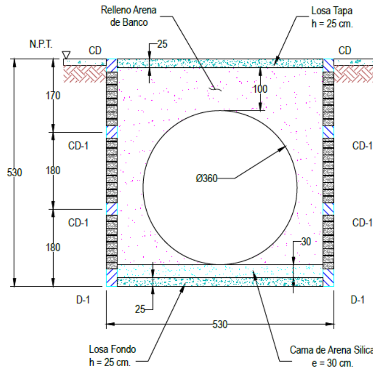
Ilustración 8. Corte longitudinal de fosa para tanques de almacenamiento.
