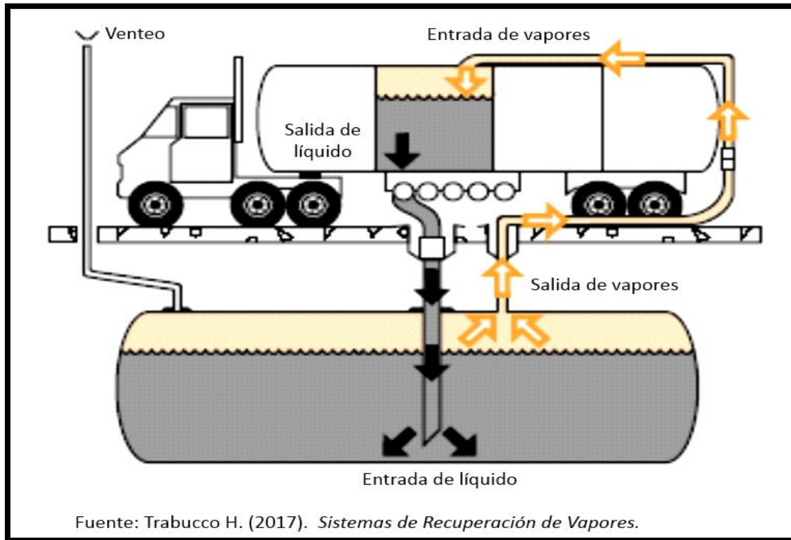
Ilustración 9. Sistema de recuperación de vapores Fase I.
