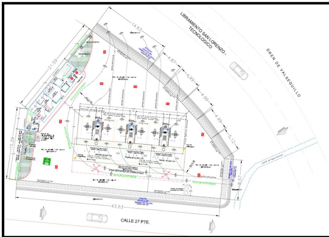
Ilustración 5. Plano arquitectónico del proyecto ARQ-01.
