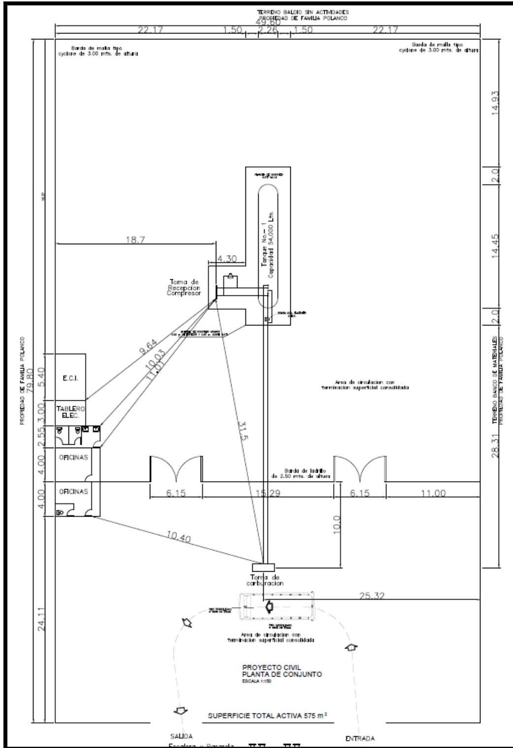
IMAGEN 6. ARREGLO GENERAL DE LA ESTACIÓN DE CARBURACIÓN (SE ANEXA PLANO).
