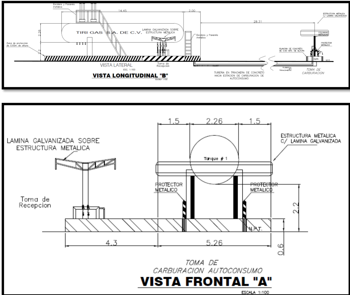
IMAGEN 7. TANQUE DE ALMACENAMIENTO QUE SE UTILIZARÁ EN LA ESTACIÓN DE CARBURACIÓN.
