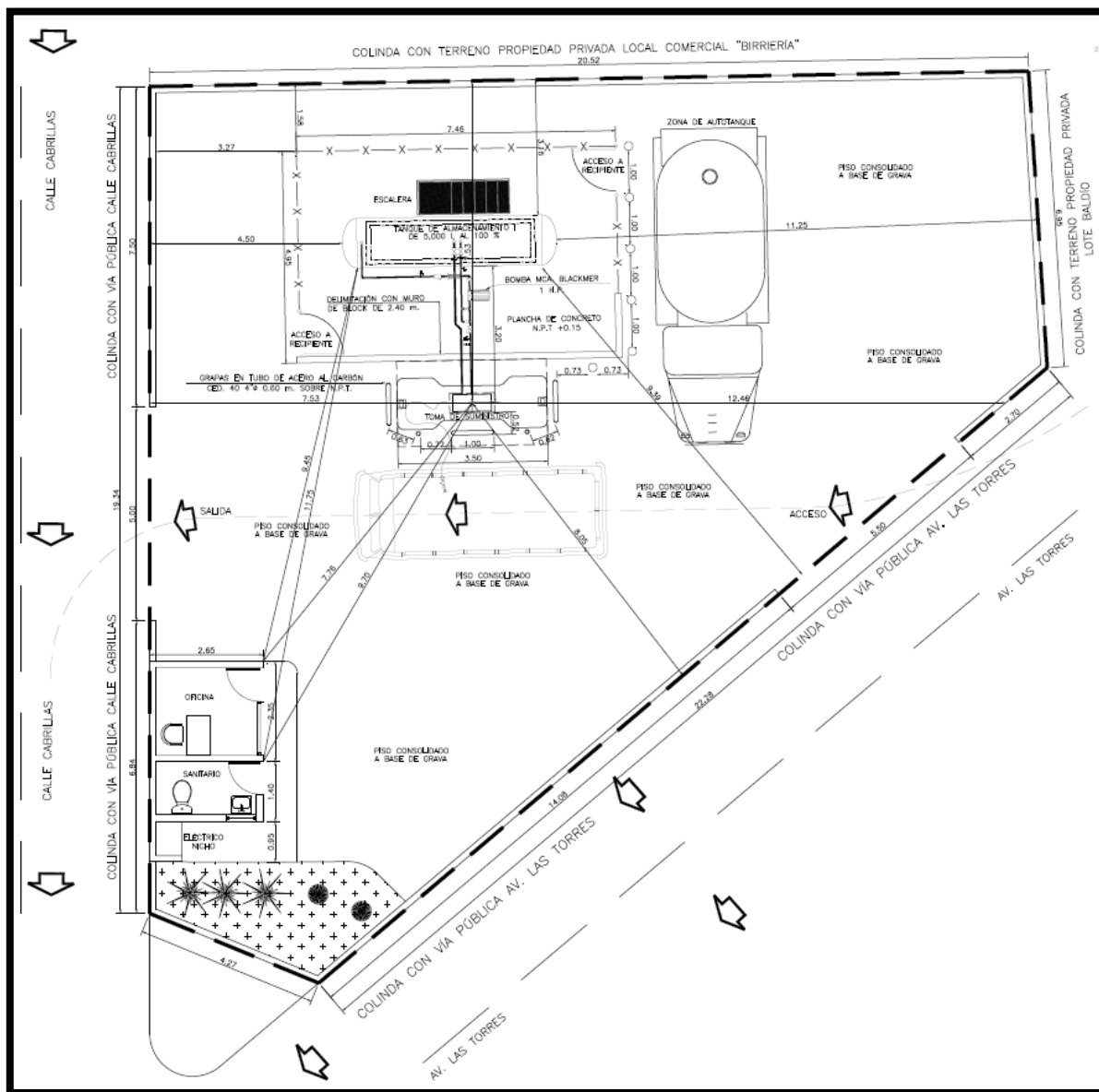
IMAGEN 7. ARREGLO GENERAL DE LA ESTACIÓN DE CARBURACIÓN (SE ANEXA PLANO).
