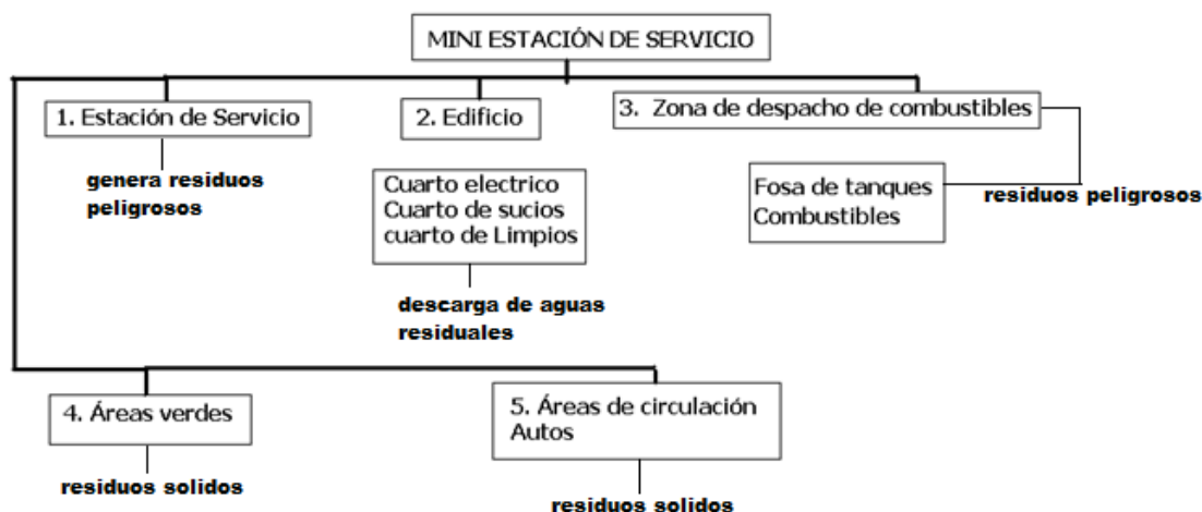
Diagrama de flujo de Operaciones
