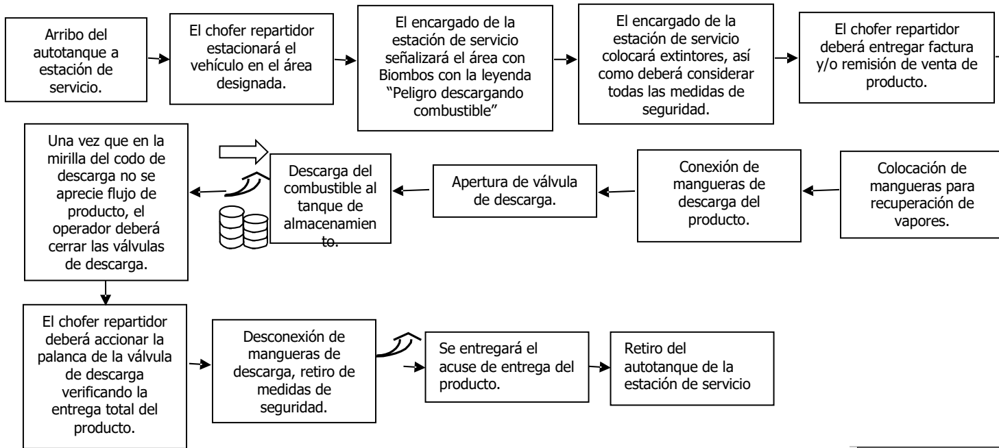
Figura III.1. Diagrama de flujo del proceso.
