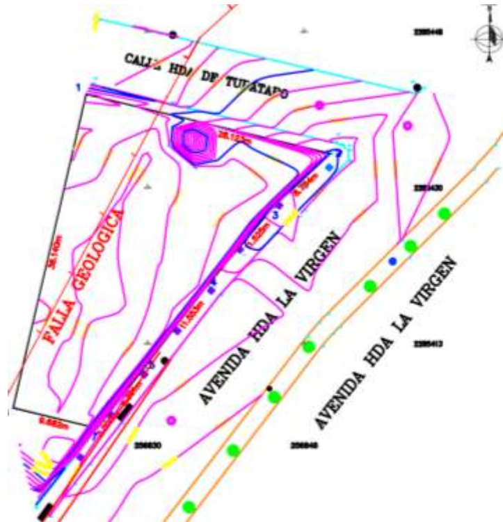
Figura III.1.b)-1 Plano Topográfico
