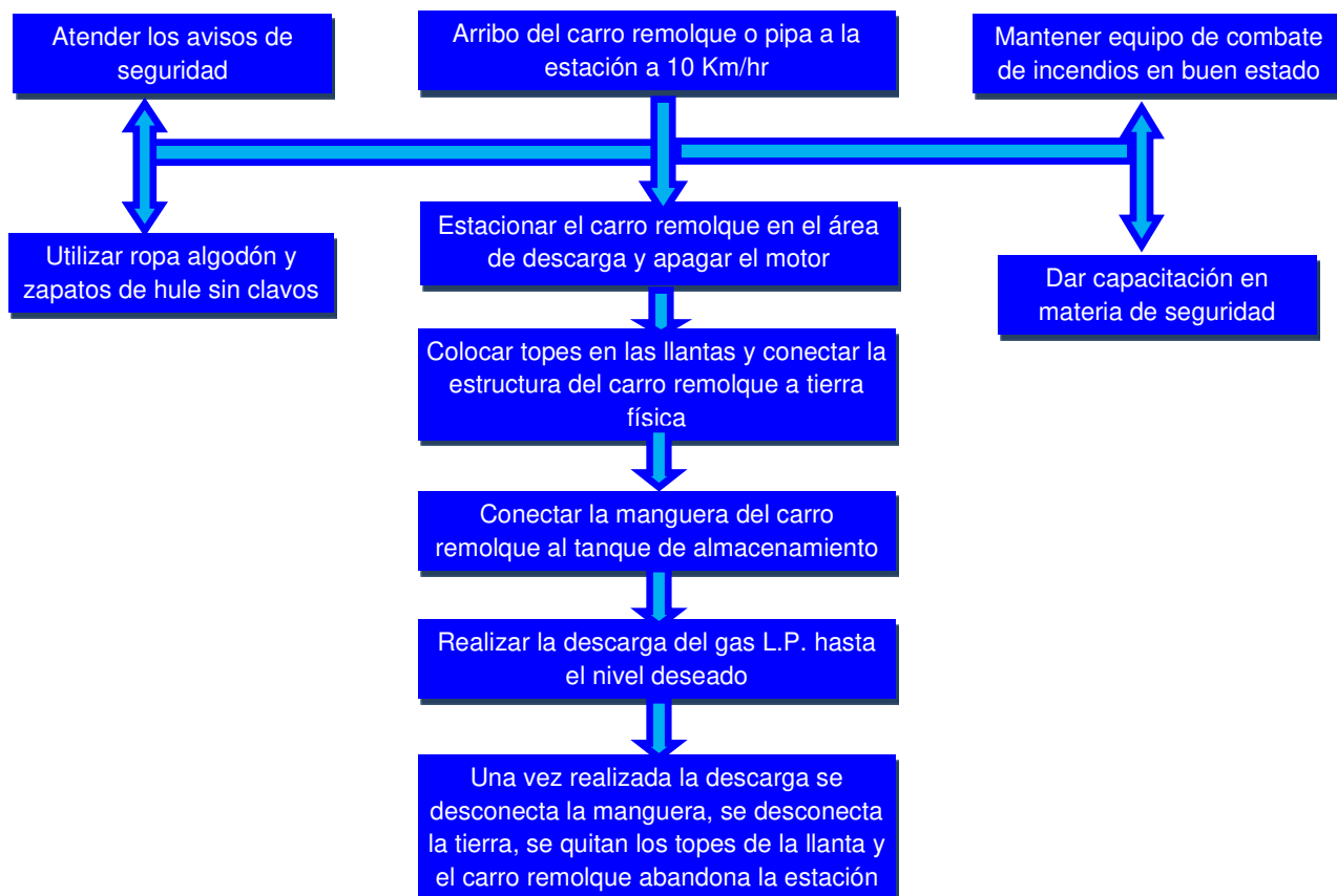
Diagrama de flujo de descarga de Gas L.P. de carro remolque al tanque de almacenamiento
