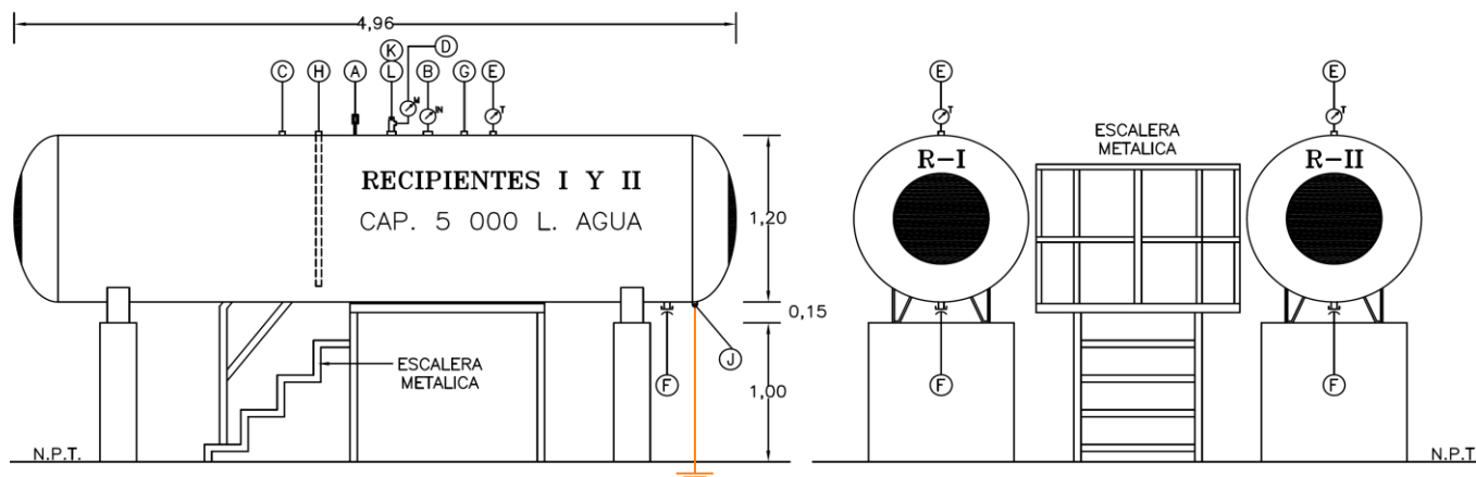
Figura 14. Instrumental de seguridad de los tanques de almacenamiento.
