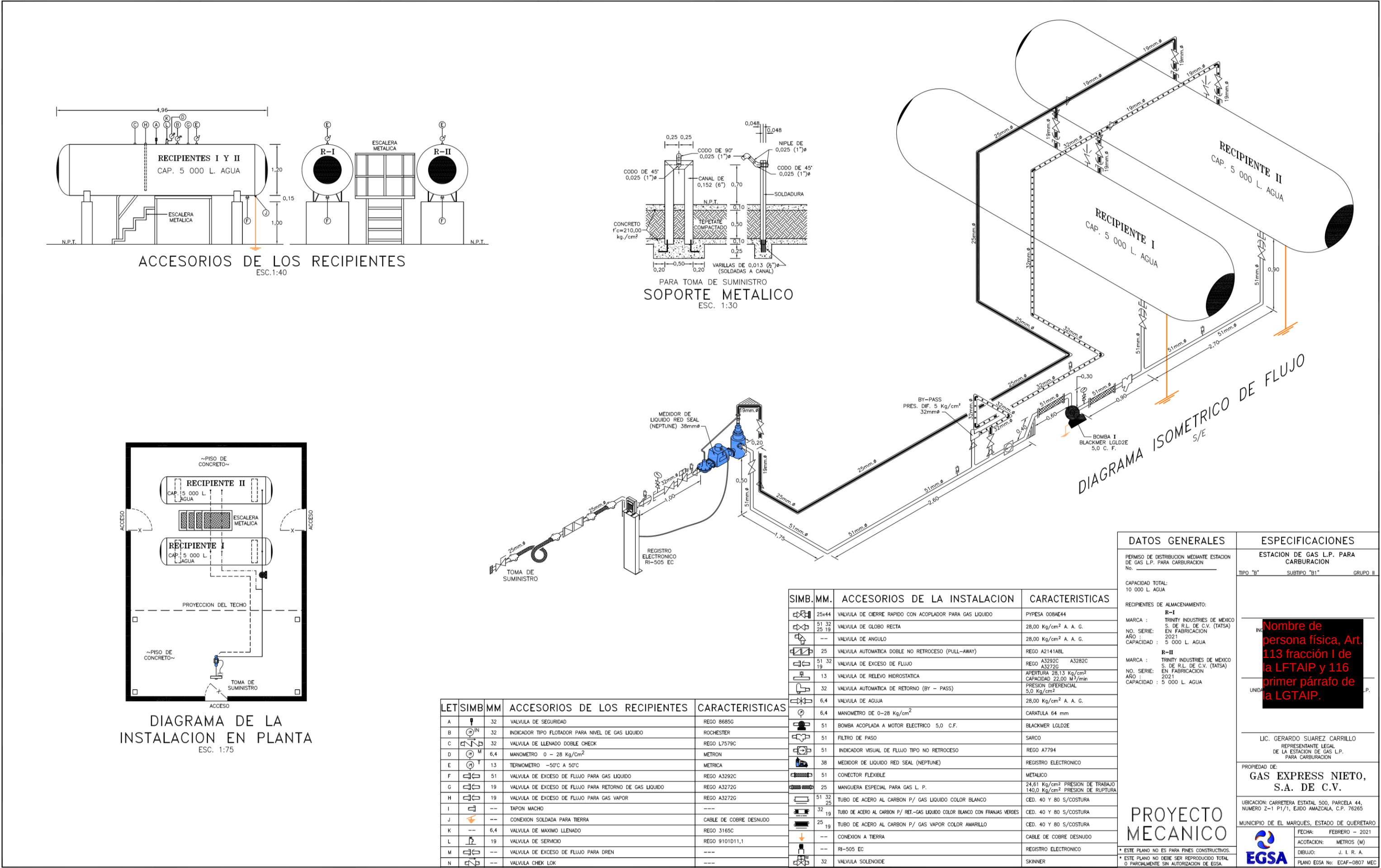
Figura 5. Plano mecánico sin escala con detalles de los tanques de almacenamiento y equipamiento de la estación proyectada.
