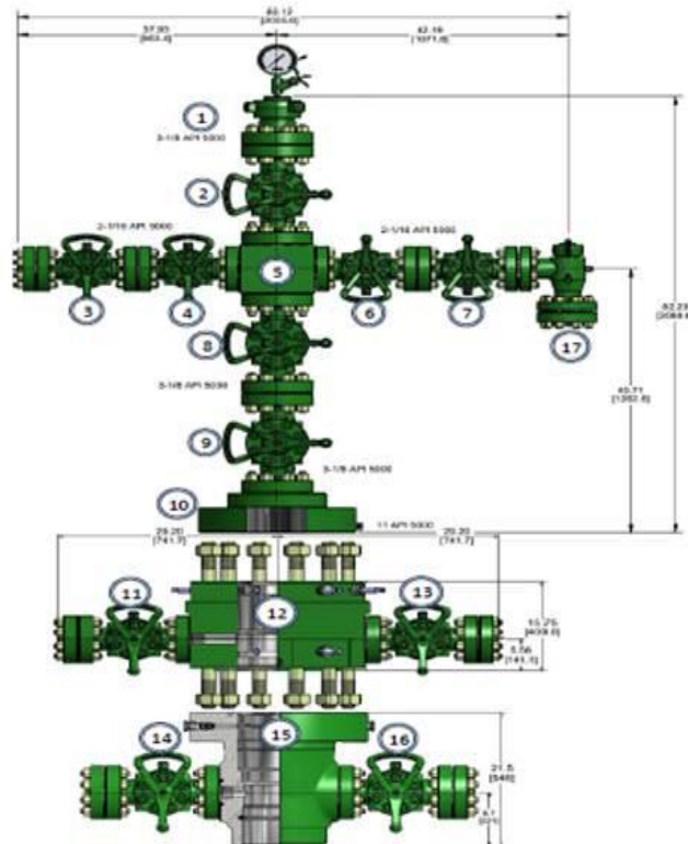
Figura 25. Arreglo preliminar de cabezales y árbol para el proyecto pozo Sakb-1EXP.
