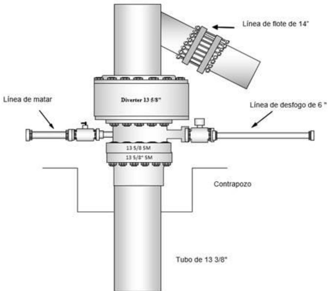
Figura 23. Arreglo del carrete de control y desviador de flujo 13 5/8" para Etapa 12 1/4"
