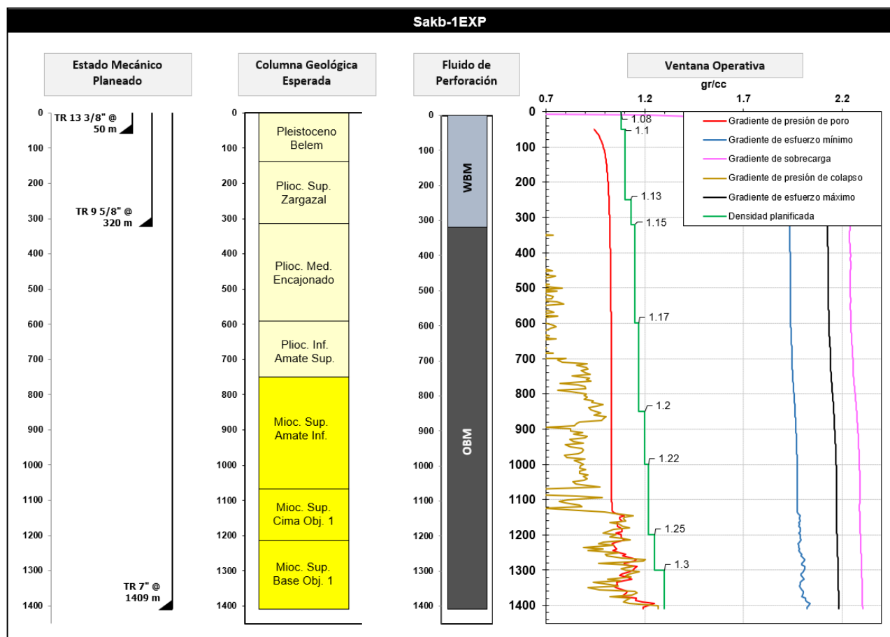
Figura 2. Estado mecánico propuesto.
