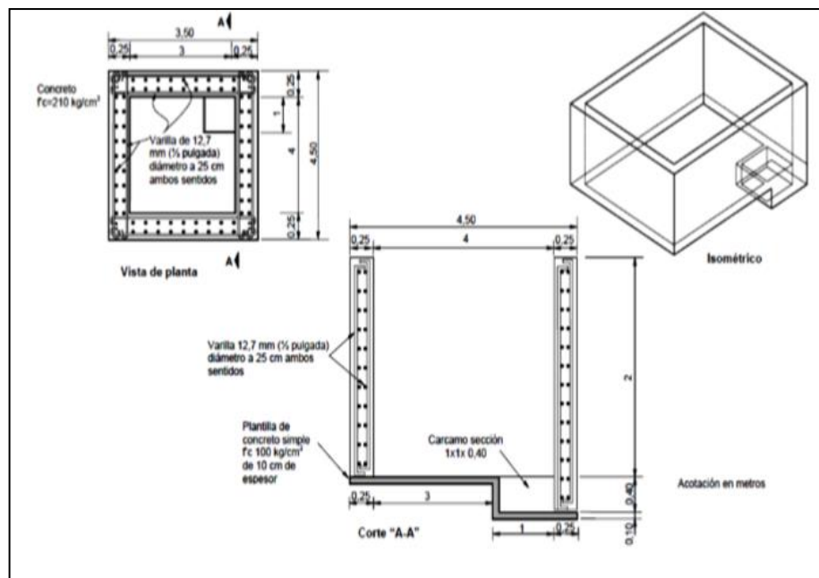
Figura 21. Diseño del contra pozo.
