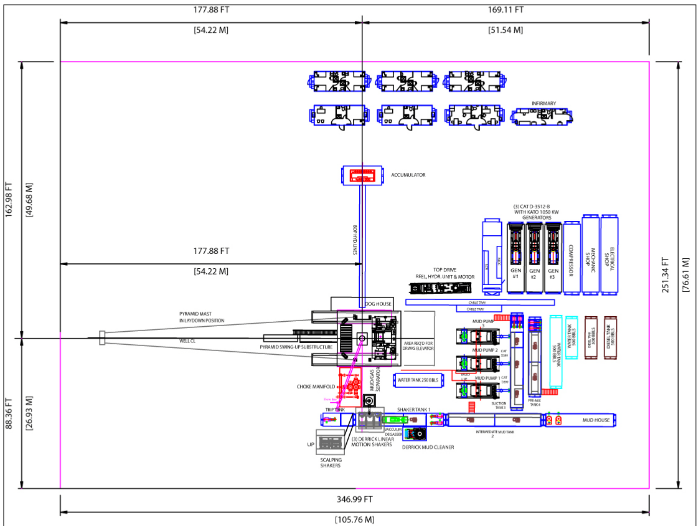
Figura 22. Diseño del arreglo de un equipo de perforación de 2.000 HP
