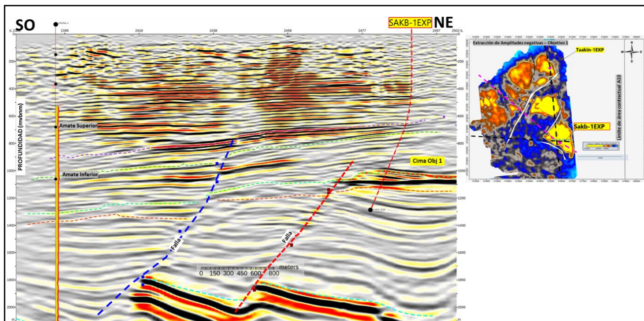
Figura 10. Sección sísmica arbitraria que atraviesa Sakb-1EXP y el pozo Otatal-1. Mapa de amplitudes del Objetivo.
