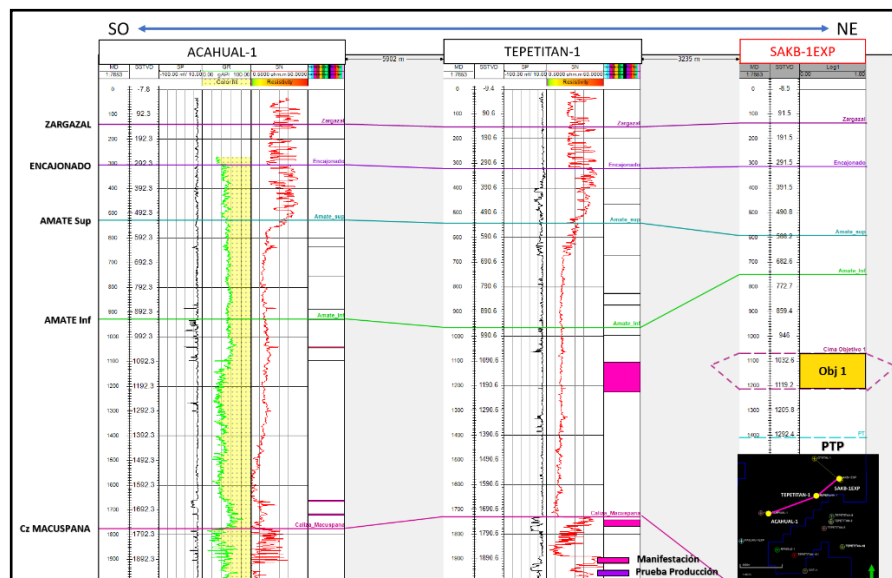
Figura 7. Correlación estructural de la localización Sakb-1EXP y sus pozos aledaños Acahual-1 y Tepetitán-1.
