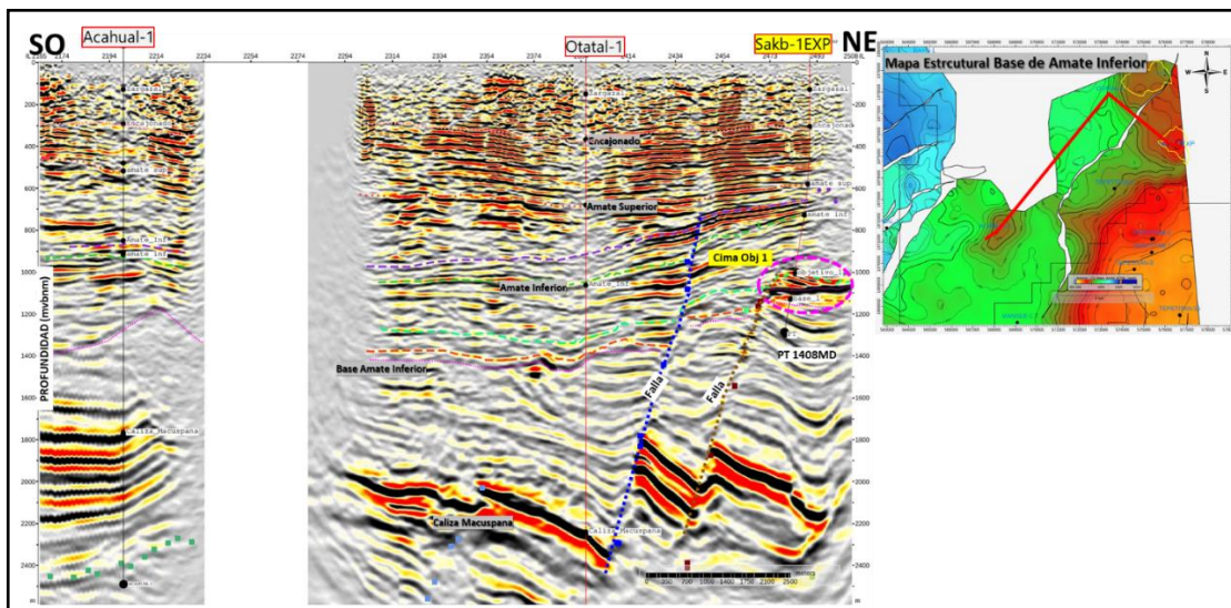
Figura 6. Ubicación estructural del pozo Sakb-1EXP y los rasgos sísmicos de la Formación Amate Inferio.
