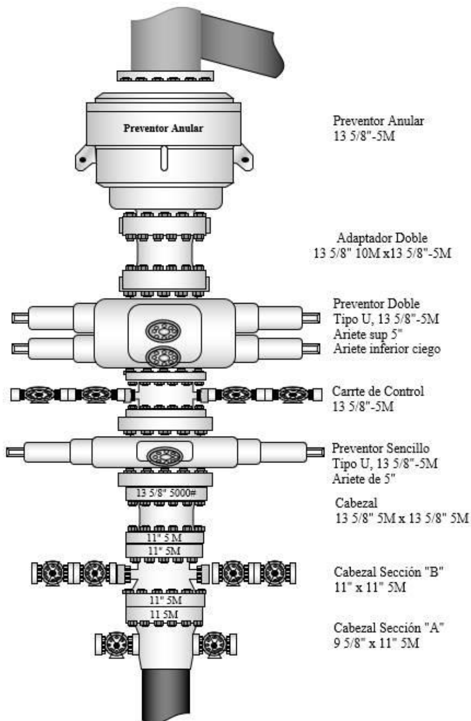
Figura 24. Arreglo 11" 5M y preventor anular 11" 5M, para la etapa 8 1/2"
