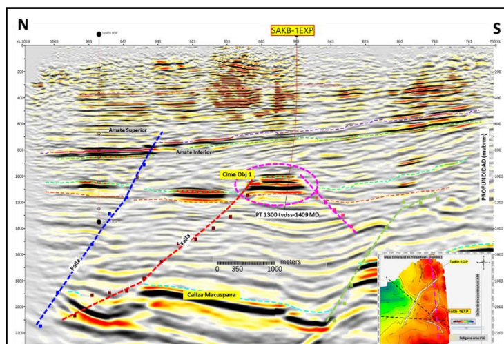
Figura 9. Sección sísmica línea arbitraria que atraviesa sobre el pozo Sakb-1EXP. Mapa estructural del Objetivo.
