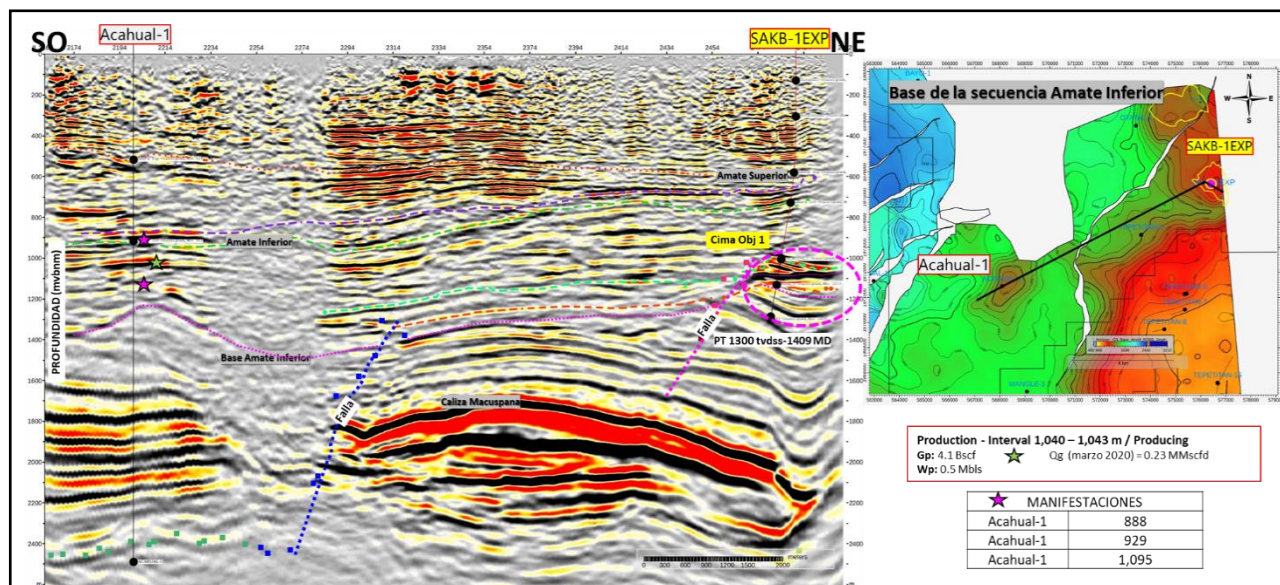
Figura 8. Línea sísmica arbitraria entre Acahual-1 y Sakb-1EXP. Mapa estructural en profundidad de base de Amate inferior.
