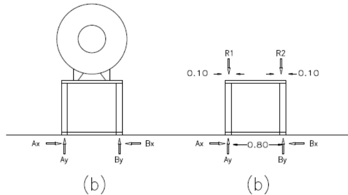
DIAGRAMA DE CUERPO LIBRE SIN ESC.
