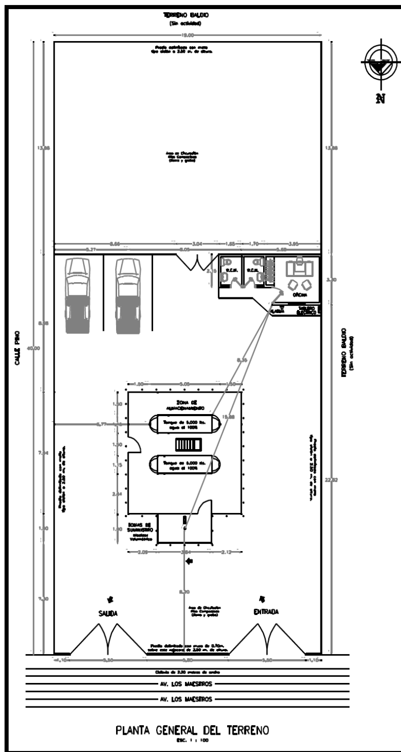
IMAGEN 7. ARREGLO GENERAL DE LA ESTACIÓN DE CARBURACIÓN (SE ANEXA PLANO).
