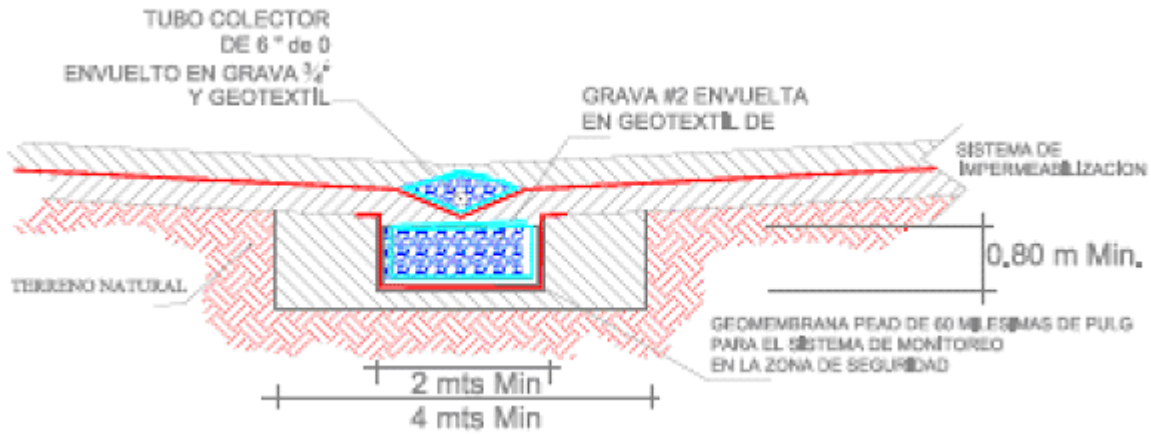
Figura A.2.1 Vista frontal del sistema de captación y extracción secundario
