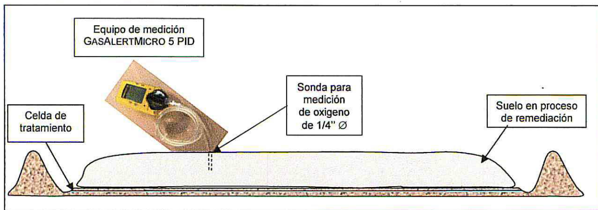
Figura 2.- Determinación de oxígeno en el proceso de tratamiento.
