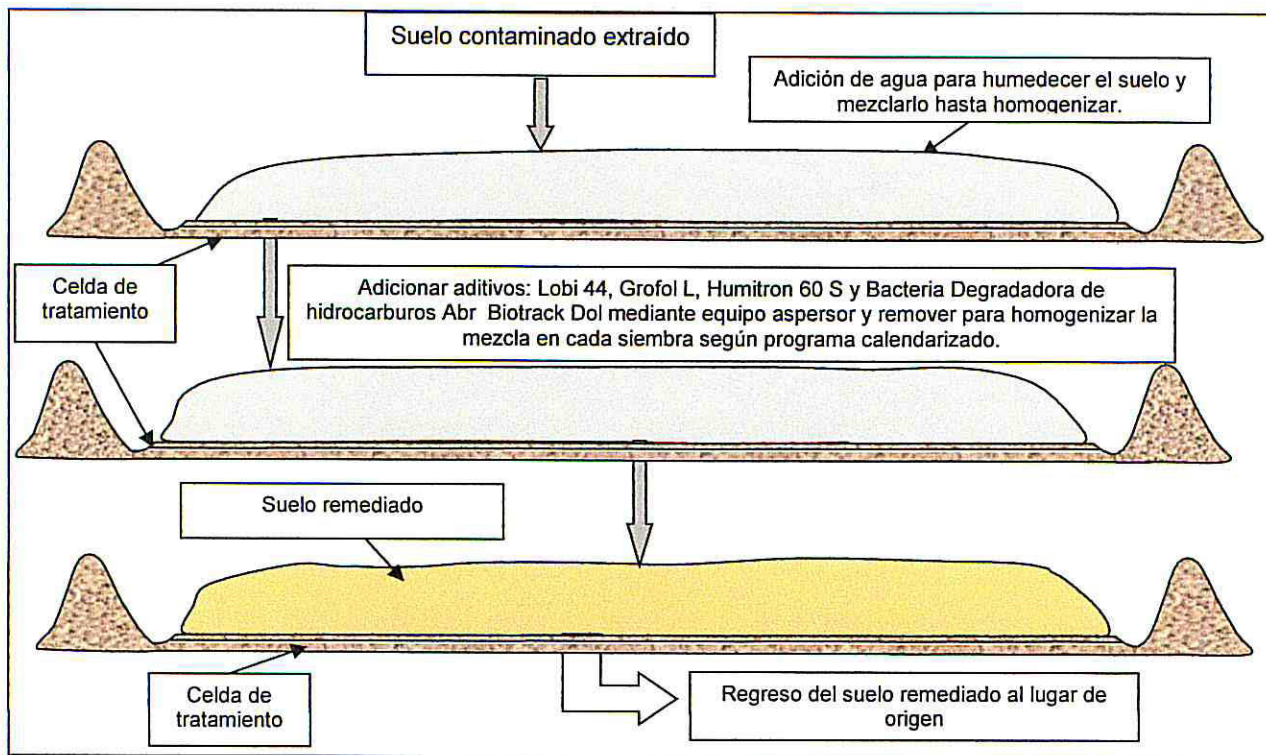
Figura 1.- Diagrama de remediación del suelo contaminado.
