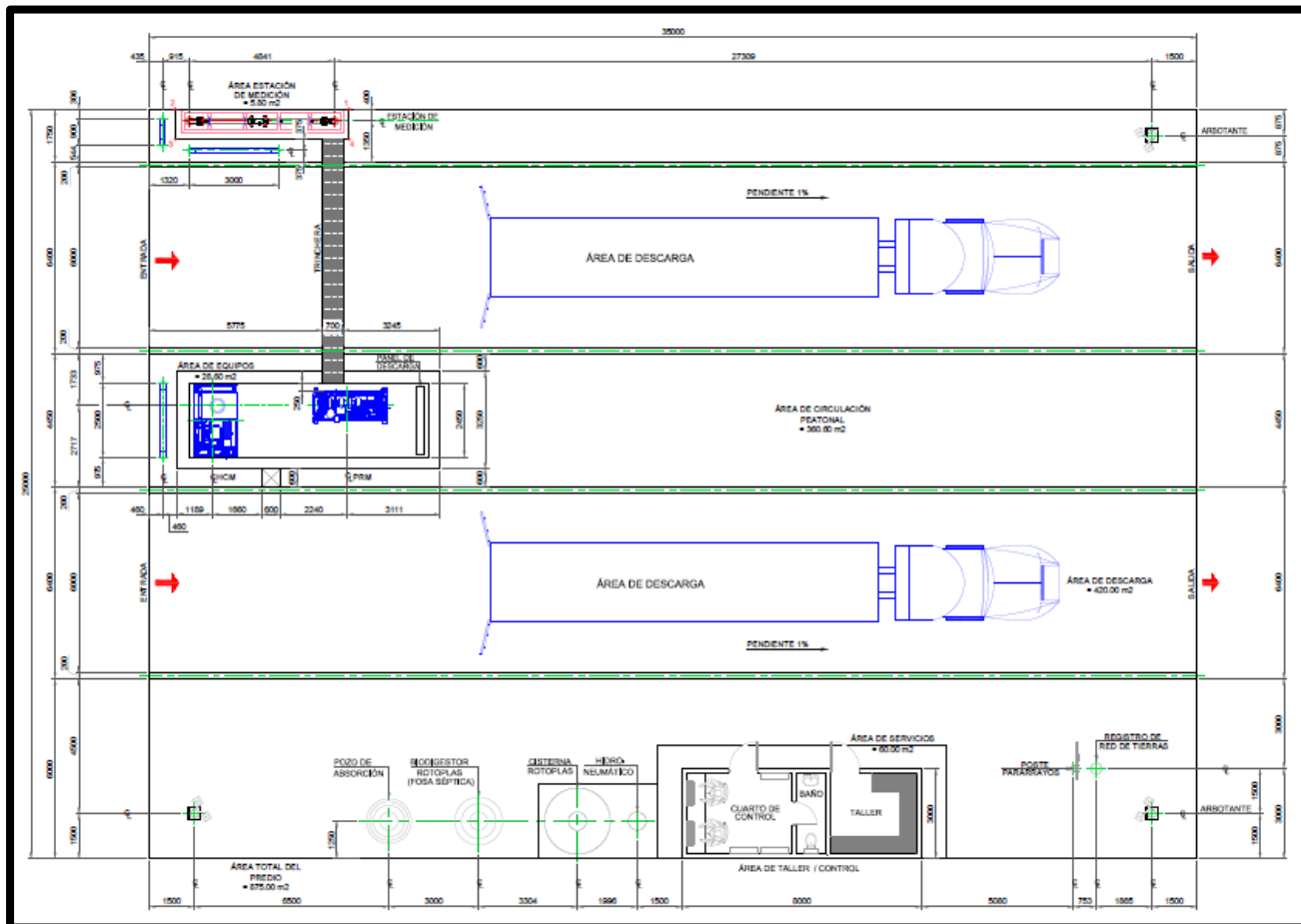
Figura 1. Plano de arreglo general de la Estación de Descompresión Celulosa y Corrugados.
