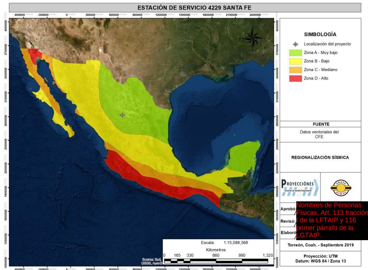
Figura 6. Regionalización sísmica.
