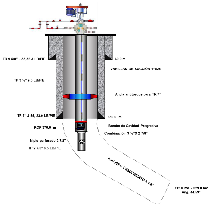
Imagen III.5. Estado mecánico propuesto
