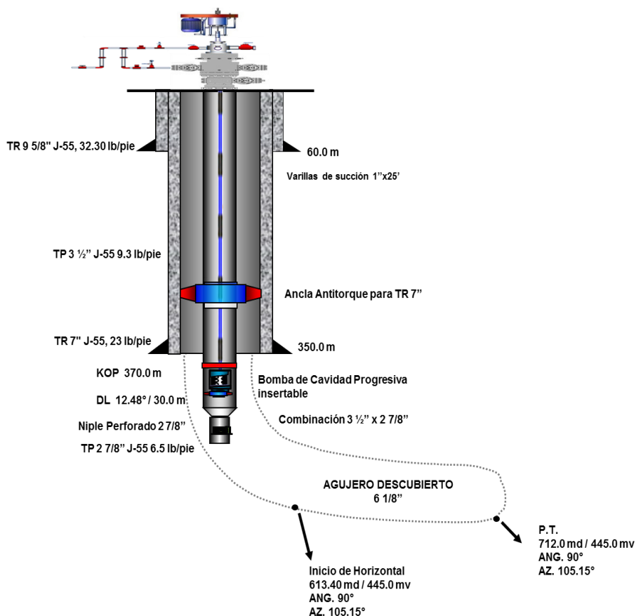
Imagen III.5. Estado mecánico propuesto
