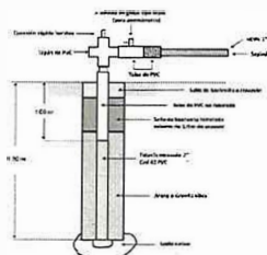
Figura Ilustrativa No. 3.2. Diseño de pozos.
