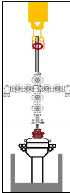
Figura 11. Fase de desmantelado de medio árbol de producción 2 1/16" 3M.
