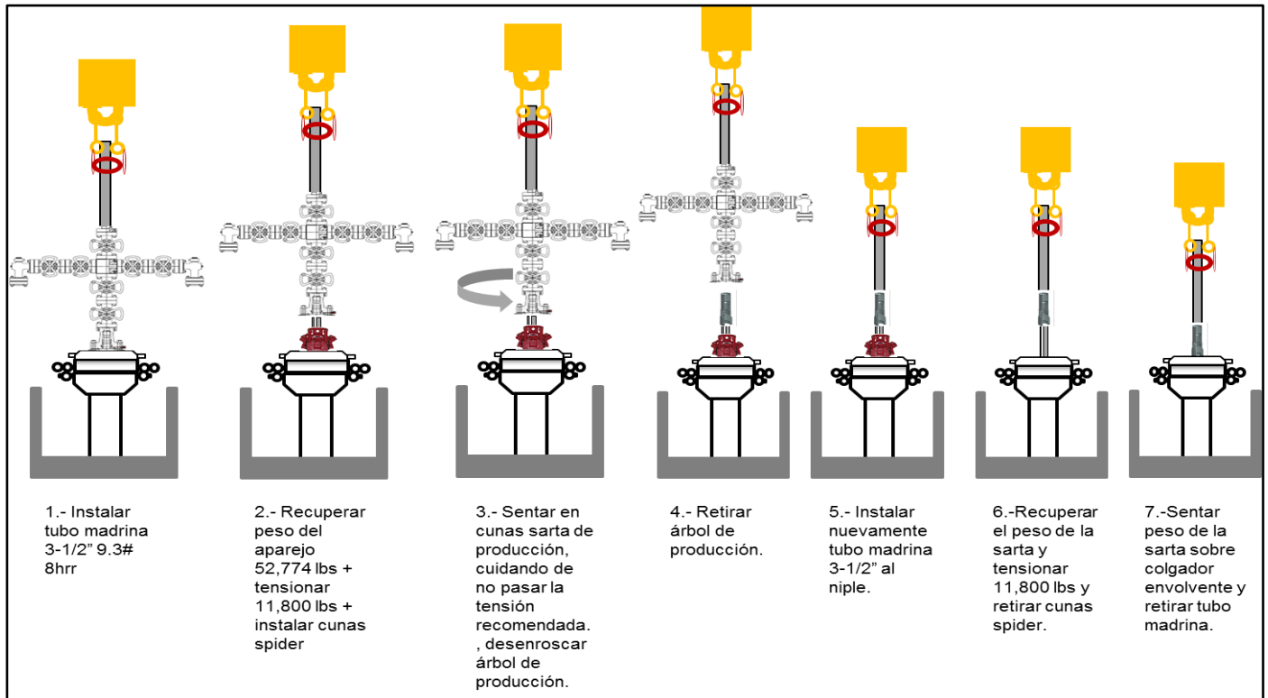
Figura 12. Fase de desmantelamiento de medio árbol de producción 2 1/16" 3M
