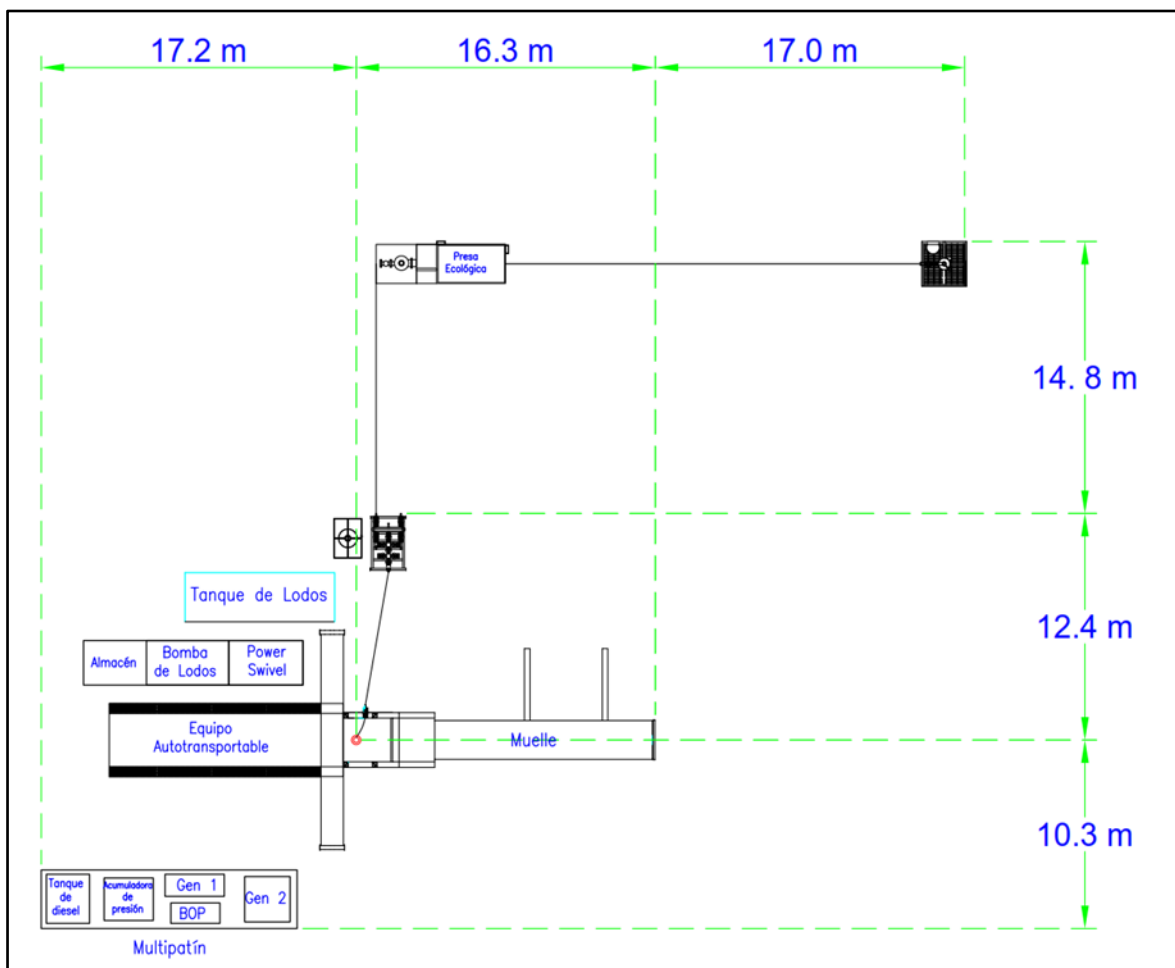
Figura 13. Diagrama de Distribución
