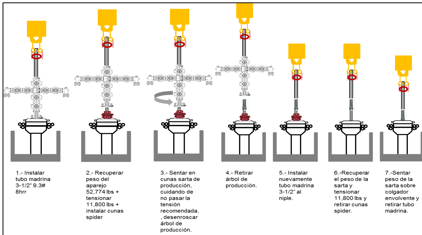
Figura 12. Fase de desmantelado de medio árbol de producción 2 1/16" 3M
