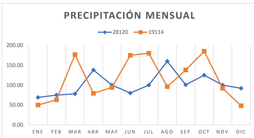
Figura 29. Precipitación mensual
