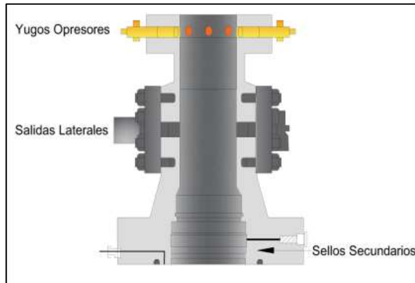
Figura 12.Cabezal de producción
