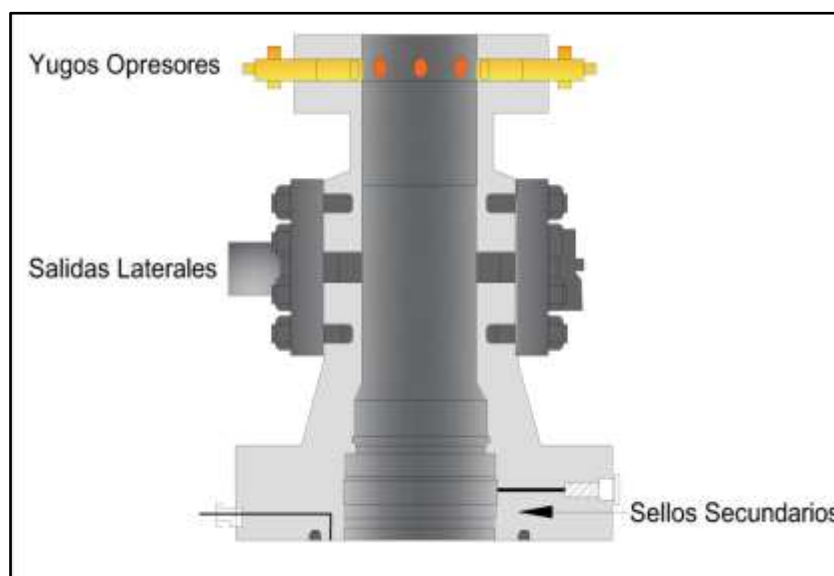
Figura 12.Cabezal de producción
