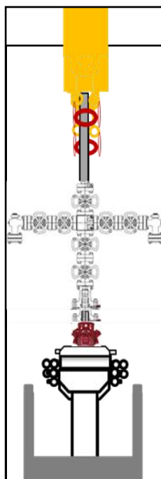
Figura 11. Fase de desmantelamiento de medio árbol de producción 2 1/16" 3M
