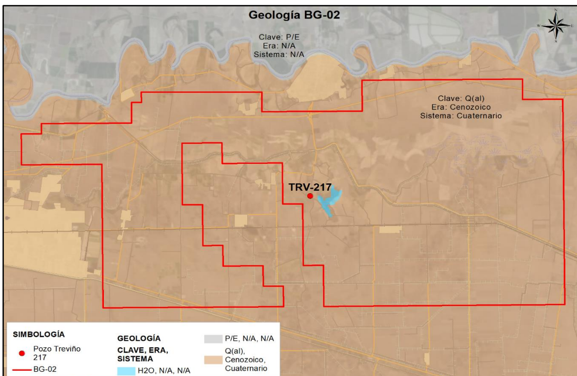
Figura 30. Geología del Área de Influencia
