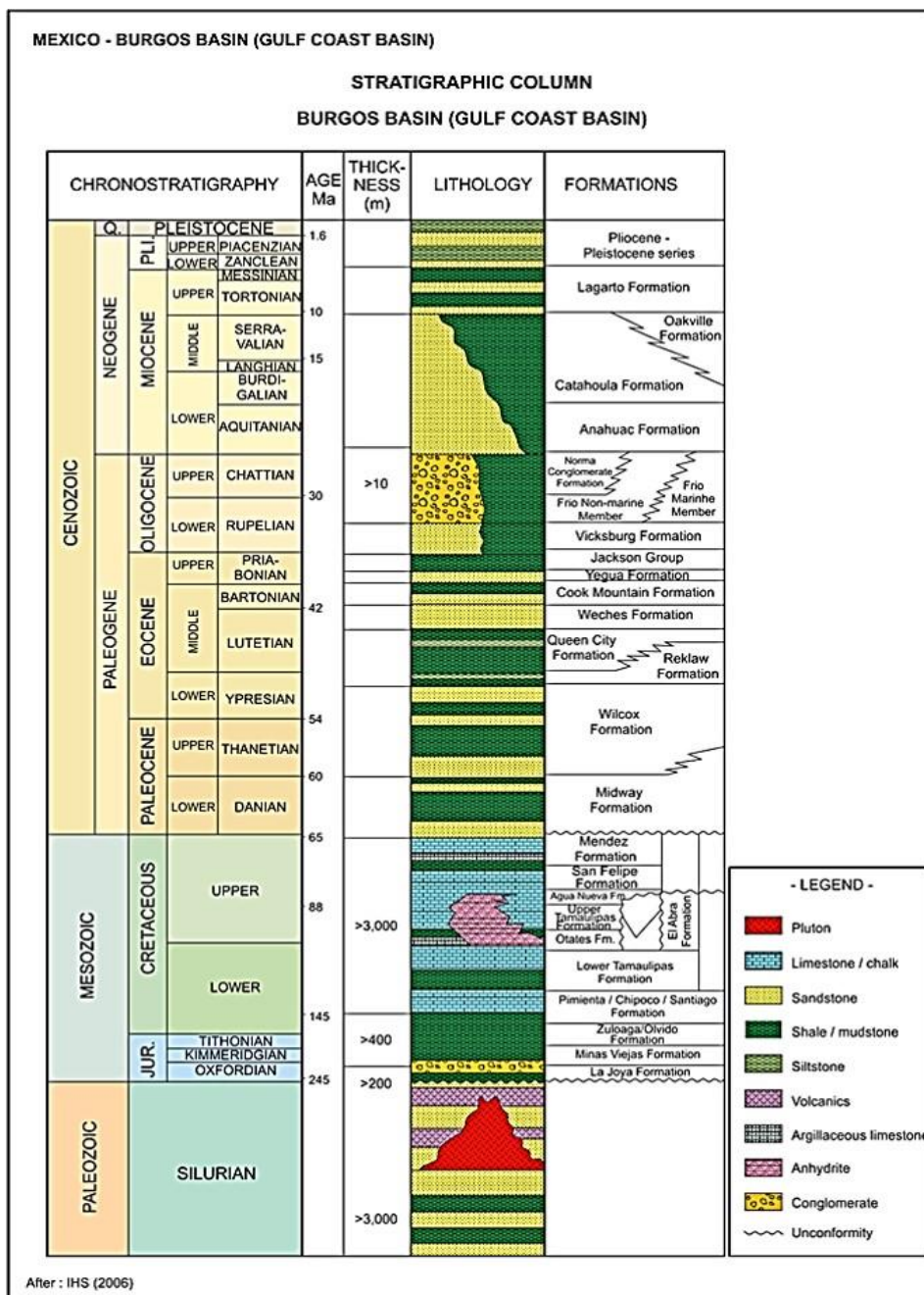
Figura 31. Columna geológica correspondiente al área de influencia
