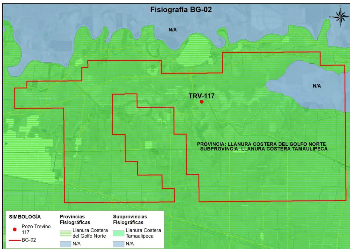
Figura 29. Fisiografía correspondiente del área de influencia.
