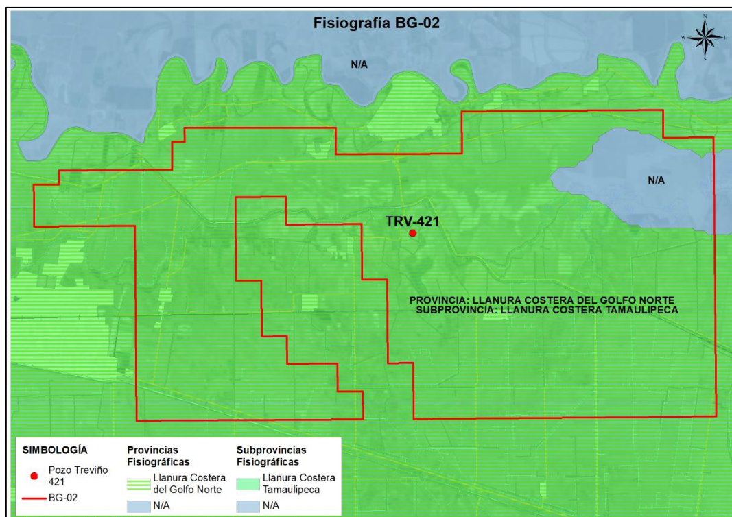
Figura 29. Fisiografía correspondiente del área de influencia.
