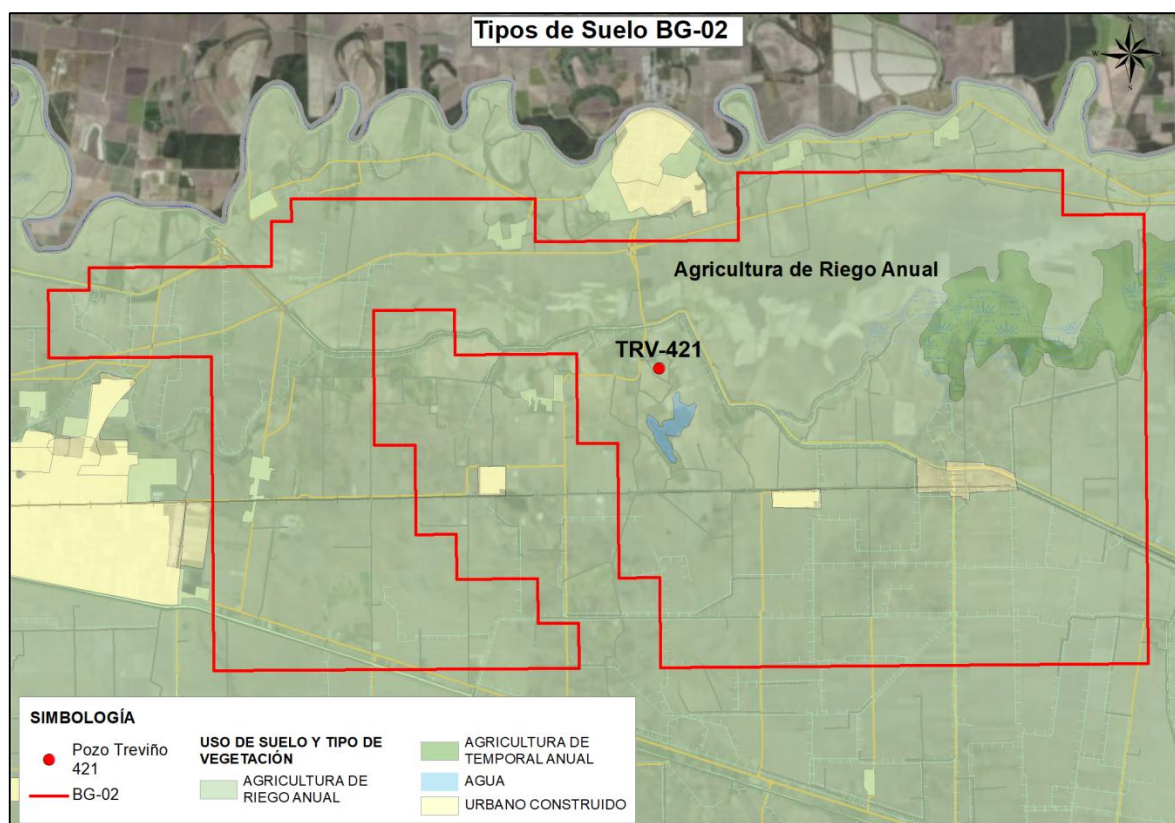
Figura 14. Uso de suelo y tipo de vegetación en el Pozo Treviño 421 en el área contractual BG-02
