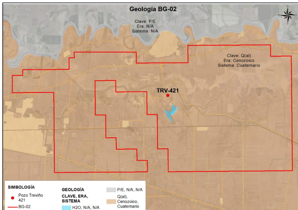
Figura 30. Geología del Área de Influencia
