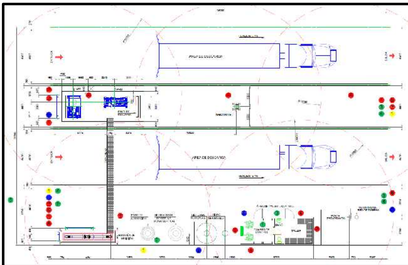
Figura 1. Ubicación de la Señalética contemplada en la Estación de Descompresión Ensenada.
