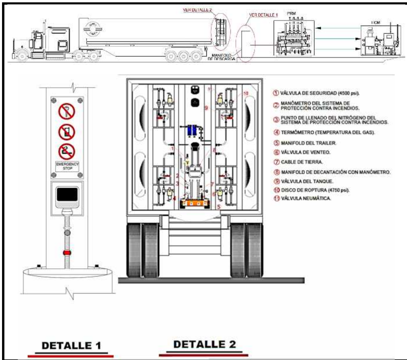
Figura 7. Equipos principales que conformarán la Estación de Descompresión Ensenada.
