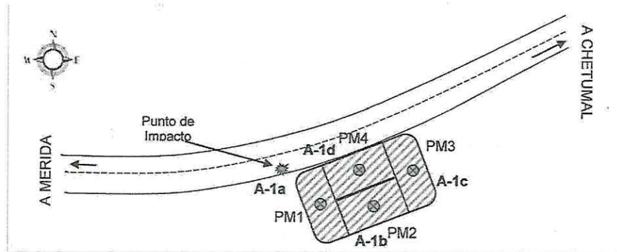
Figura 6. Ubicación de puntos del MFC propuestos.
