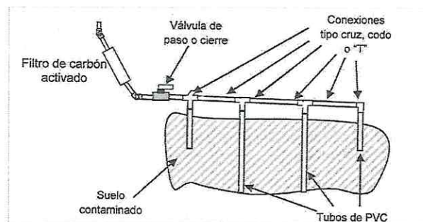
Figura 5. Filtro de carbón activado
