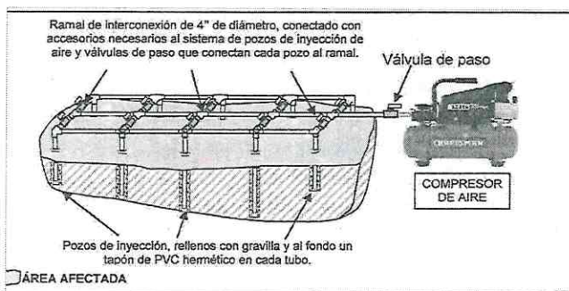
Figura 3. Red de inyección de aire
