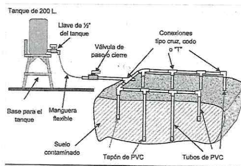
Figura 4. Infiltración de insumos
