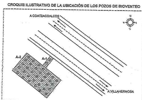
Figura 2. Ubicación de los pozos y vista de la red para la inyección de aire.
