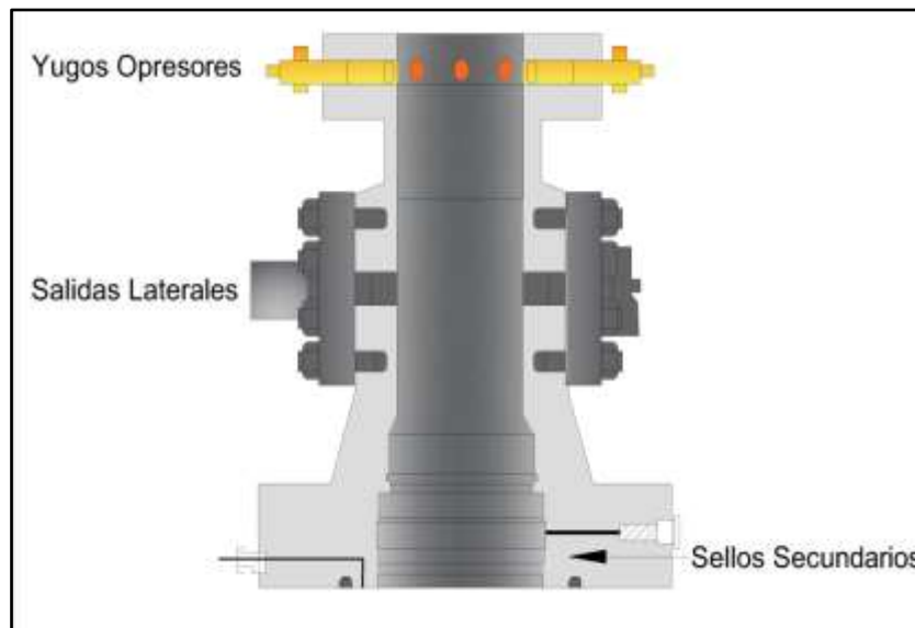
Figura 12.Cabezal de producción
