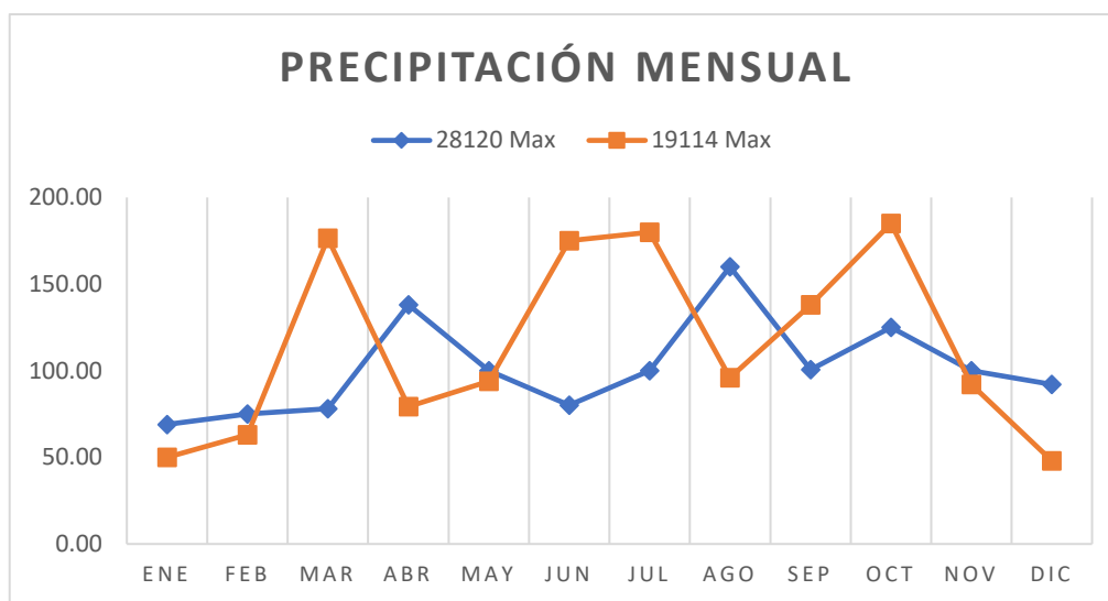
Figura 31. Precipitación mensual
