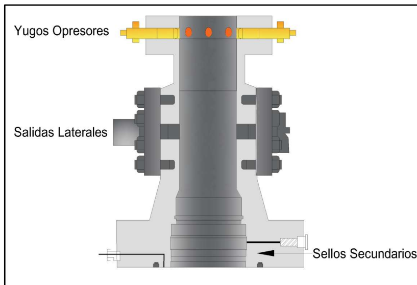
Figura 12. Cabezal de producción
