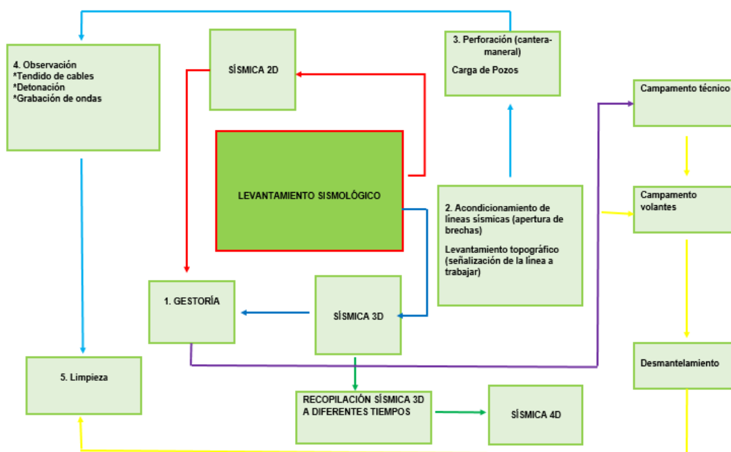
Diagrama 2. Actividades que conforman a las prospecciones sismológicas.
