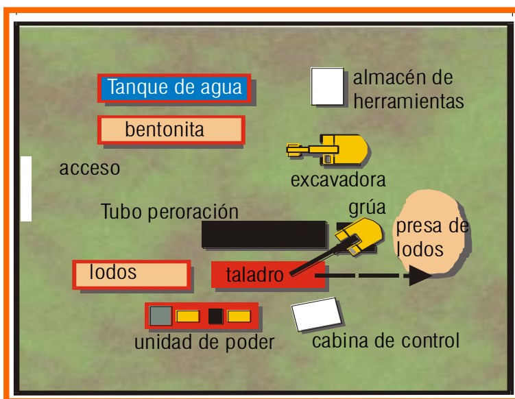
Figura 18. Acomodo del equipo para la construcción de ductos por el método de perforación horizontal direccional controlado.
