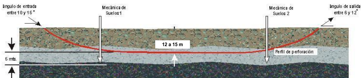
Figura 19. Perfil de perforación.
