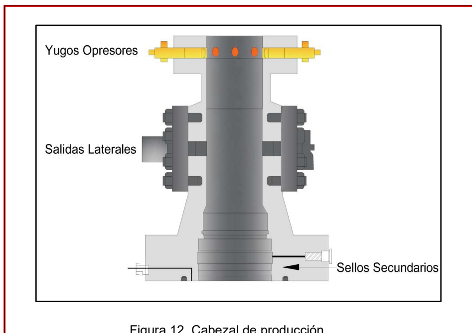
Figura 12. Cabezal de producción
