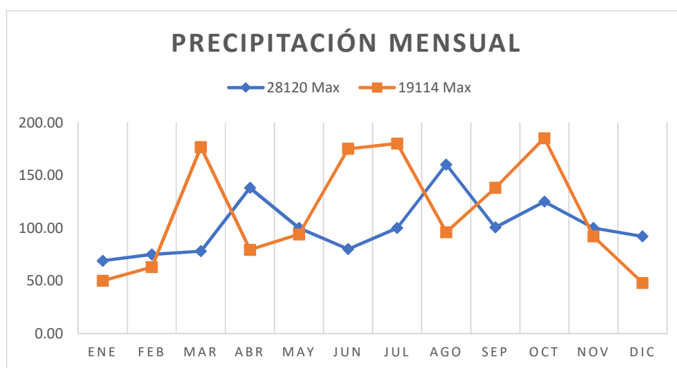
Figura 31. Precipitación mensual
