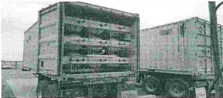
Interior de uno de los cinco contenedores tipo semirremolque donde se aprecian equipos tipo tanques cilíndricos.
