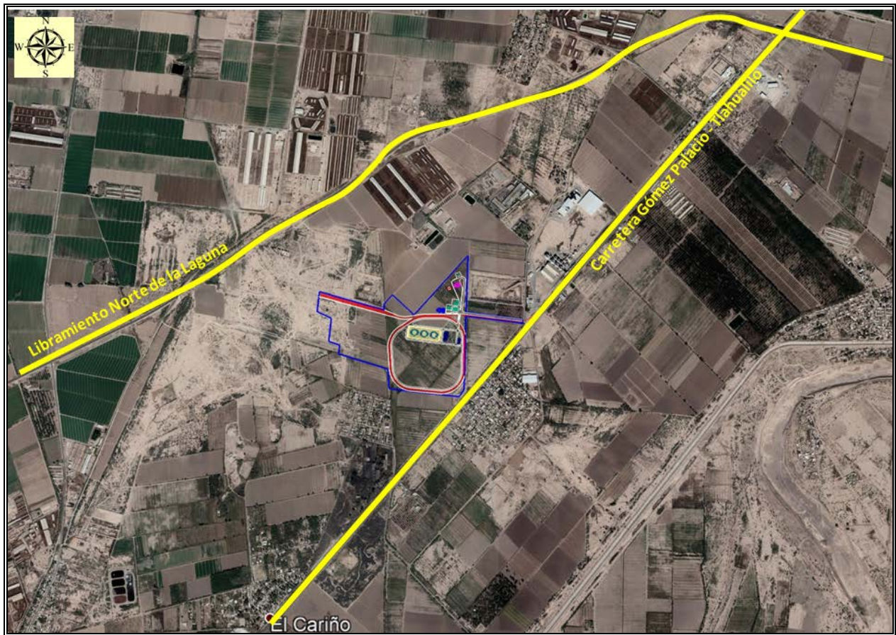
Figura II. 6 Ubicación de los accesos al predio de la TAS.
