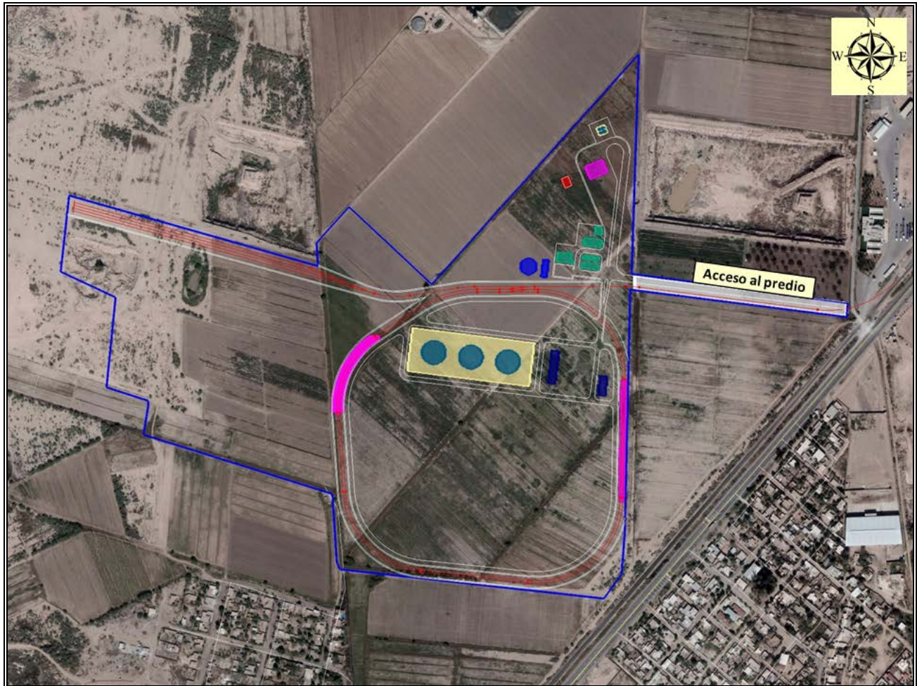
Figura II. 4 Arreglo general de la TAS Laguna.
