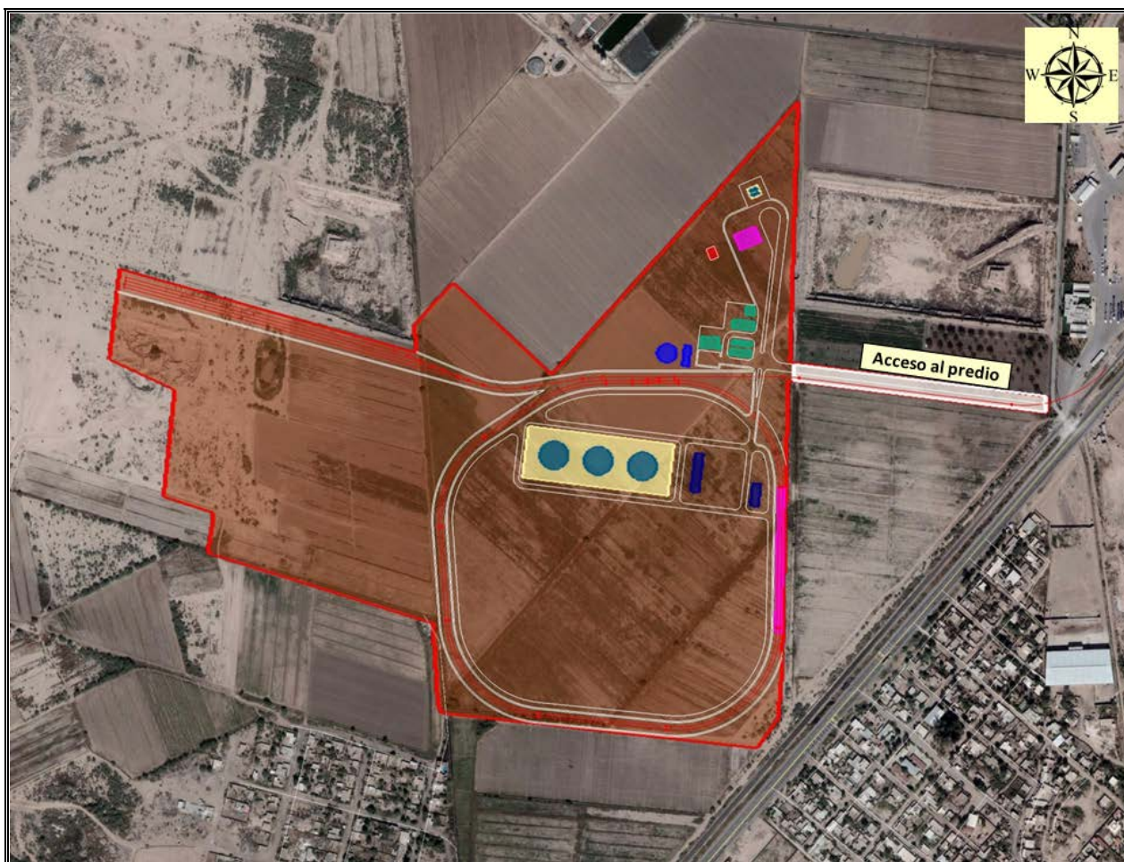
Figura I. 1 Arreglo de los Tanques para Almacenamiento de Petrolíferos.
