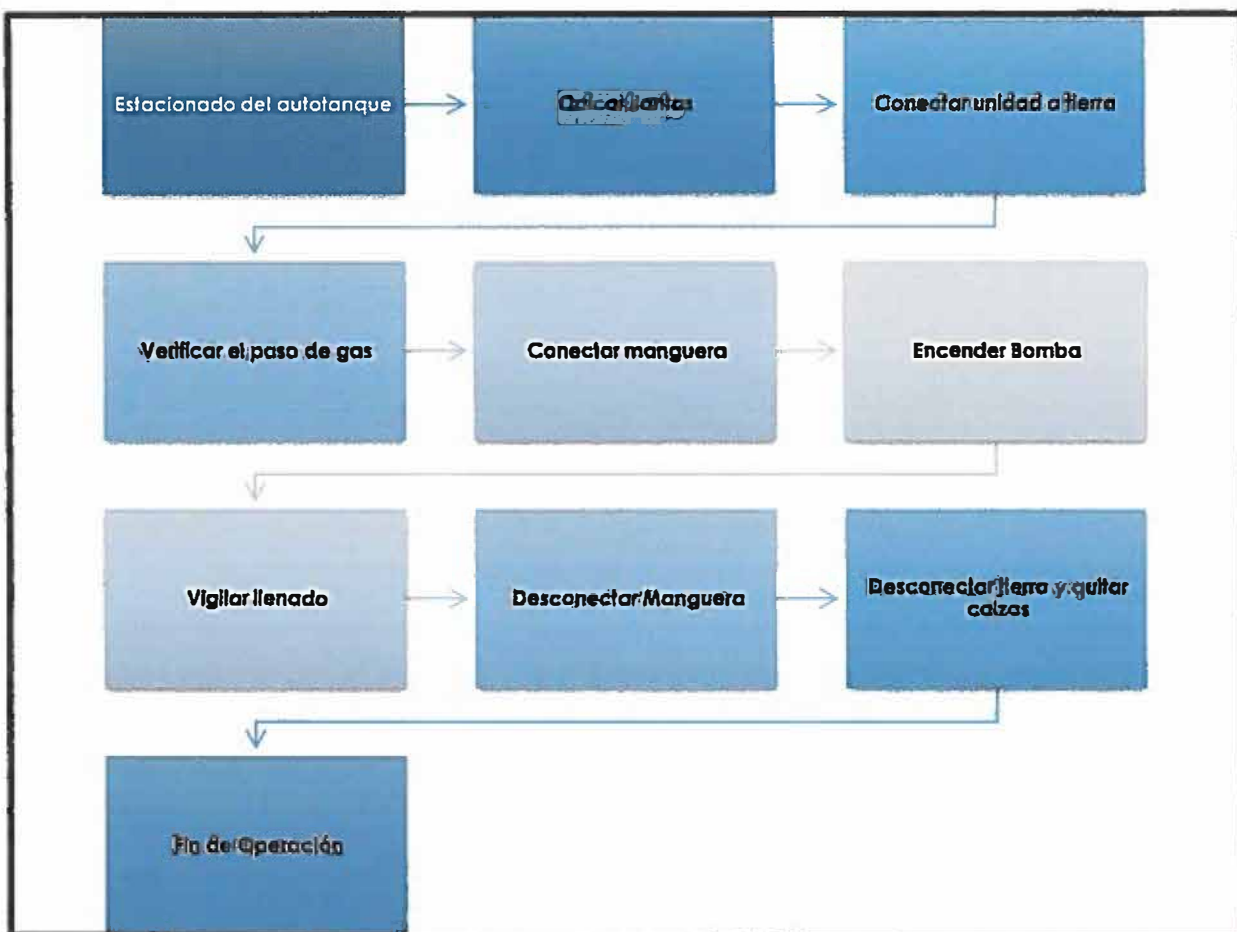
Ilustración 7. Diagrama de bloques: Para el llenado de tanques de almacenamiento
