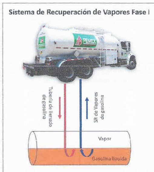
Figura 3: Sistema de Recuperación de Vapores Fase I
