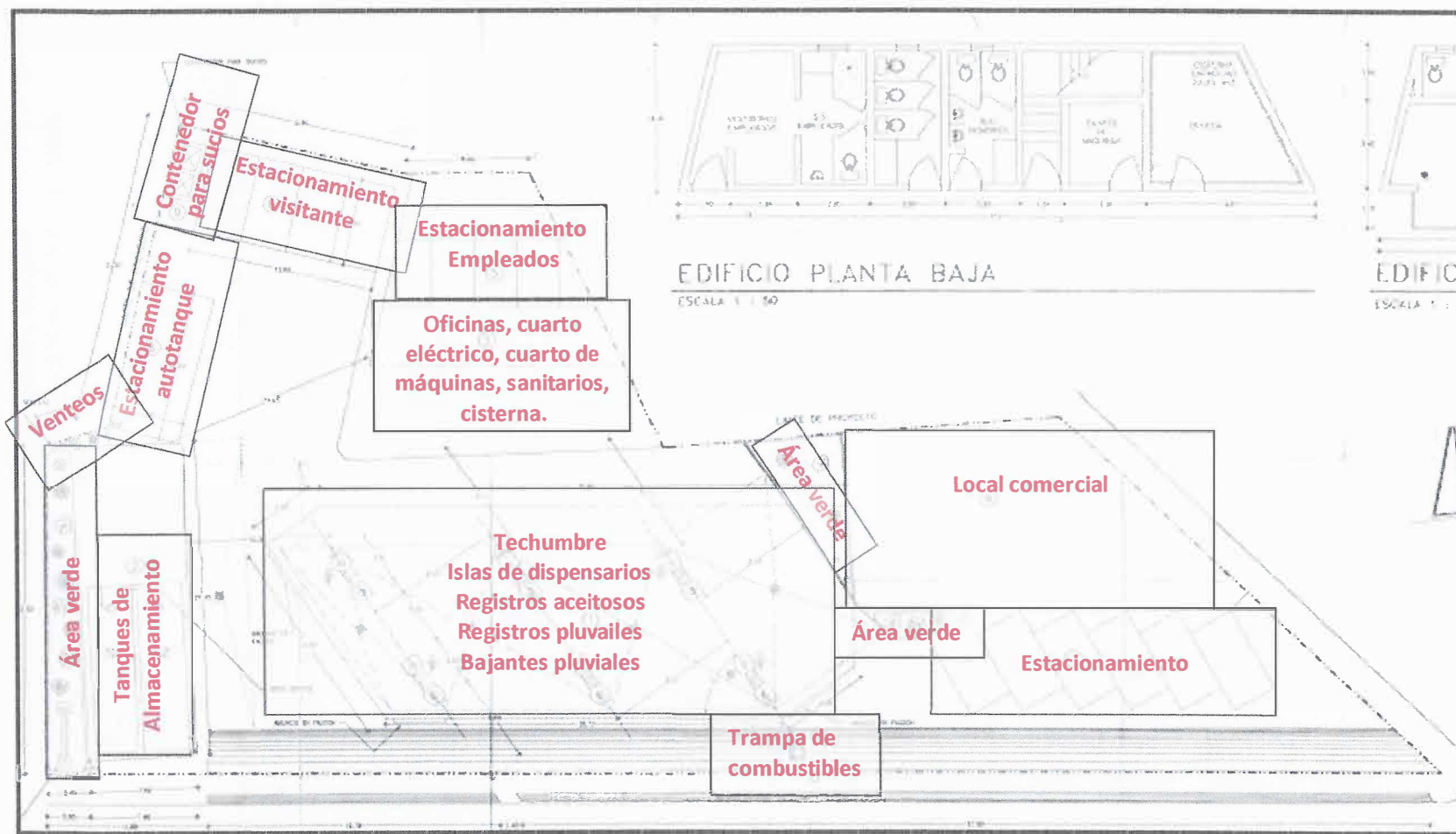
Diagrama general de la estación de servicio.
