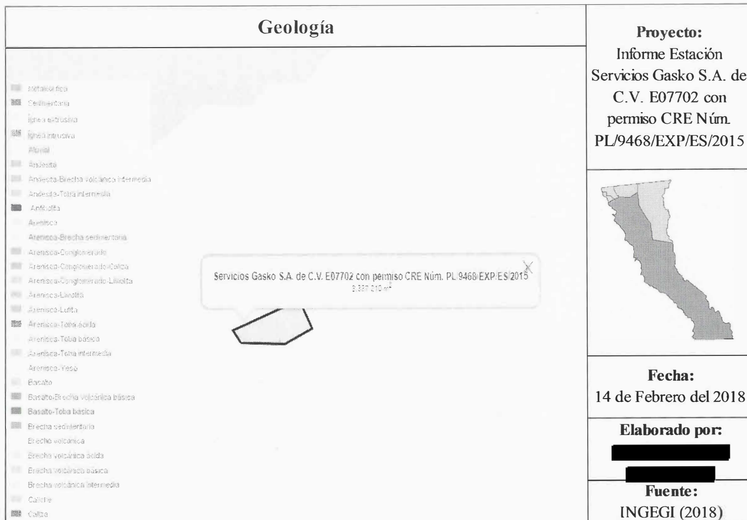
Figura 15. Geología
