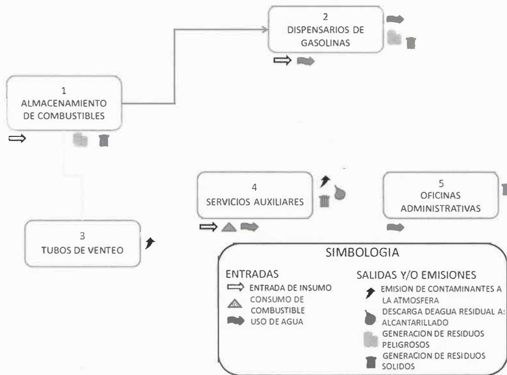
FIGURA 9. DIAGRAMA DE ALMACENAMIENTO
